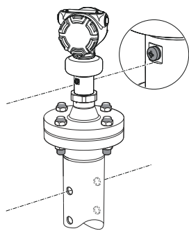
Figura 4-2: Tubo tranquilizador
