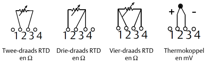
Figuur 3-1: Sensoraansluitingen
