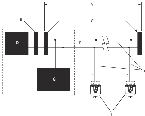
Figuur 3-3: Standaardconfiguratie voor een PROFIBUS-netwerk
