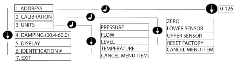
Rysunek 3-1: Schemat menu lokalnego interfejsu operatora
