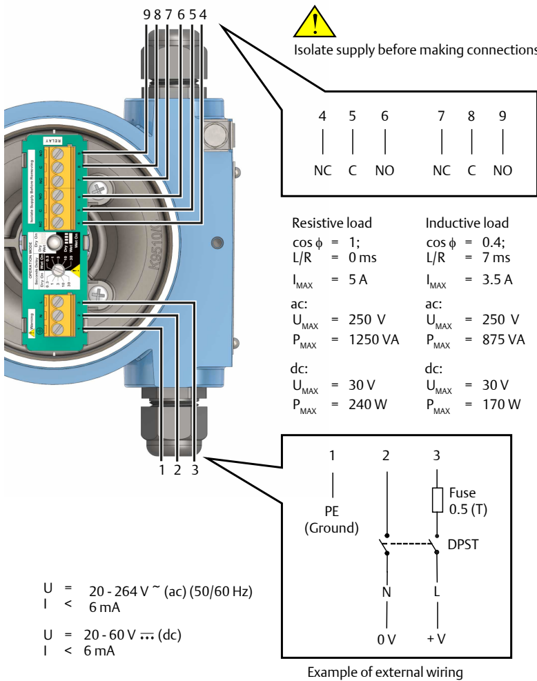
ábra 3-3: Relékimenet, DPCO (zöld címke, normál elektronikadoboz)
