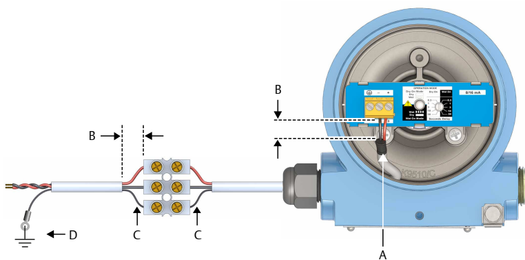
ábra 3-7: A jelkábel árnyékolásának földelése a tápellátás felőli végén
