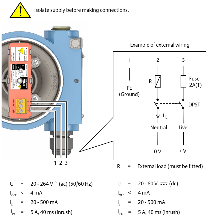
ábra 3-1: Közvetlen terhelésű, kapcsolós (kéthuzaloz, vörös címke)
