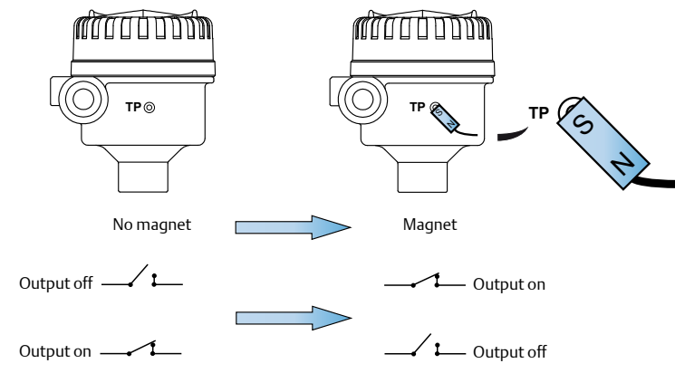
ábra 7-1: Mágneses ellenőrző pont funkció
