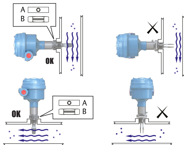
ábra 2-1: A villa helyzetének megfelelő beállítása csőbe történő szerelésnél
