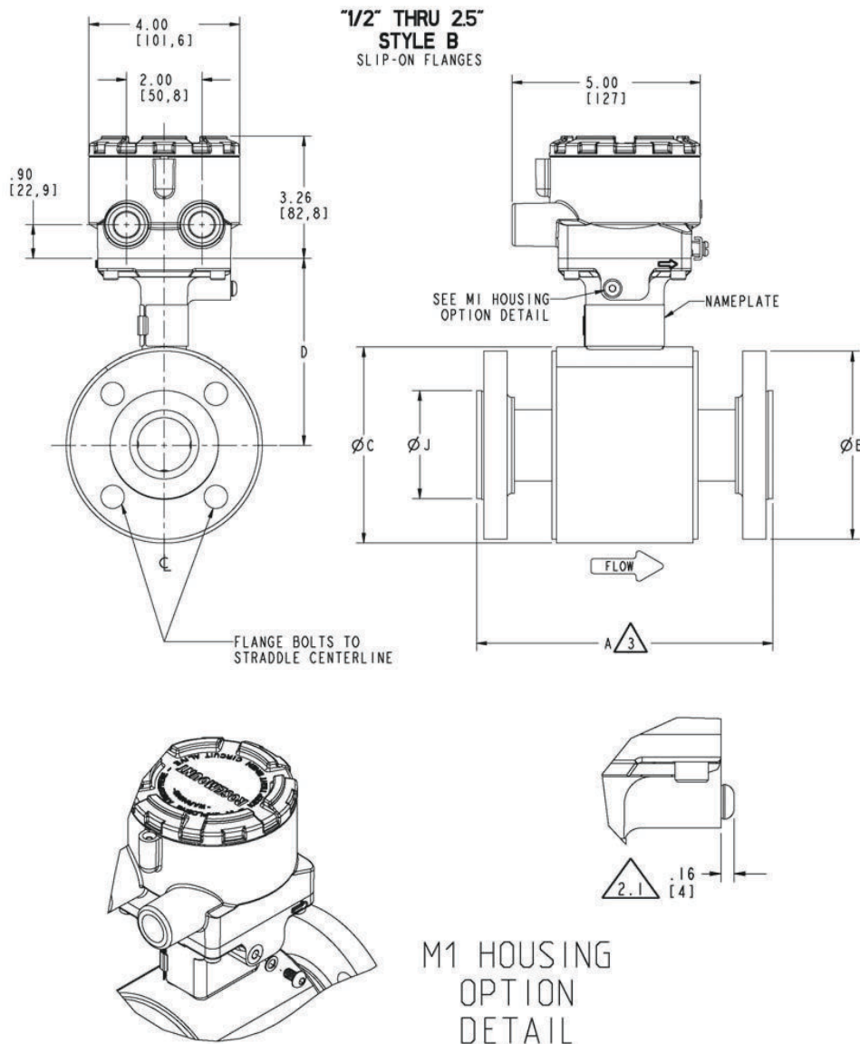
Abbildung 14: Messrohr 8705-M in Flanschbauweise 0,5 Zoll bis 2,5 Zoll (DN 15 mm bis 65 mm) Überschiebflansche - Niederdruck (P ≤ Class 300)
