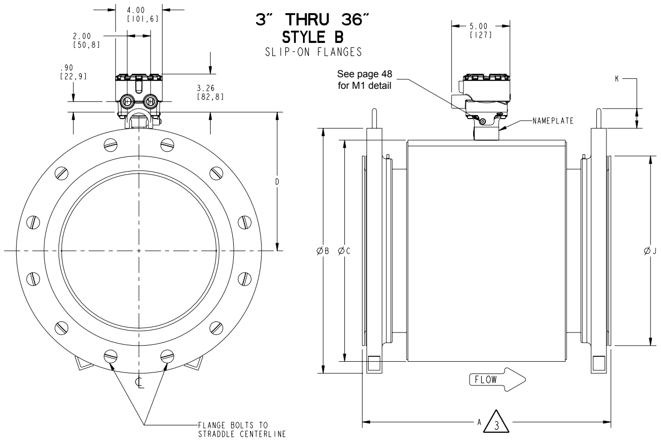
Abbildung 15: Messrohr 8705-M in Flanschbauweise 3 Zoll bis 36 Zoll (DN 80 mm bis 900 mm) Überschiebflansche - Niederdruck ( P \leq \text{Class 300} )
