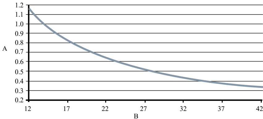
Abbildung 9: Anforderungen an den DC-Strom
