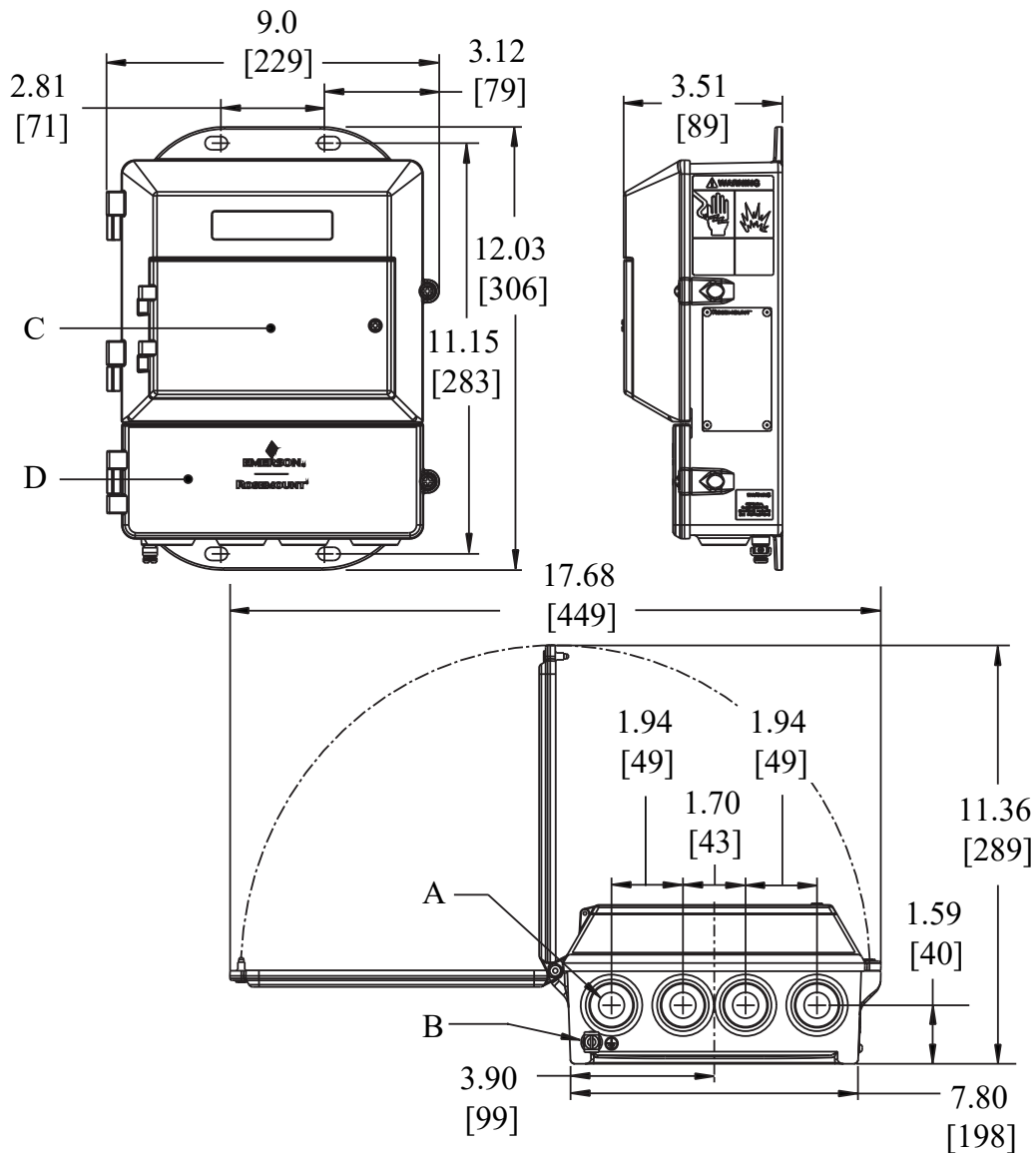
Abbildung 12: Abmessungen des Messumformers 8712 für die Wandmontage
