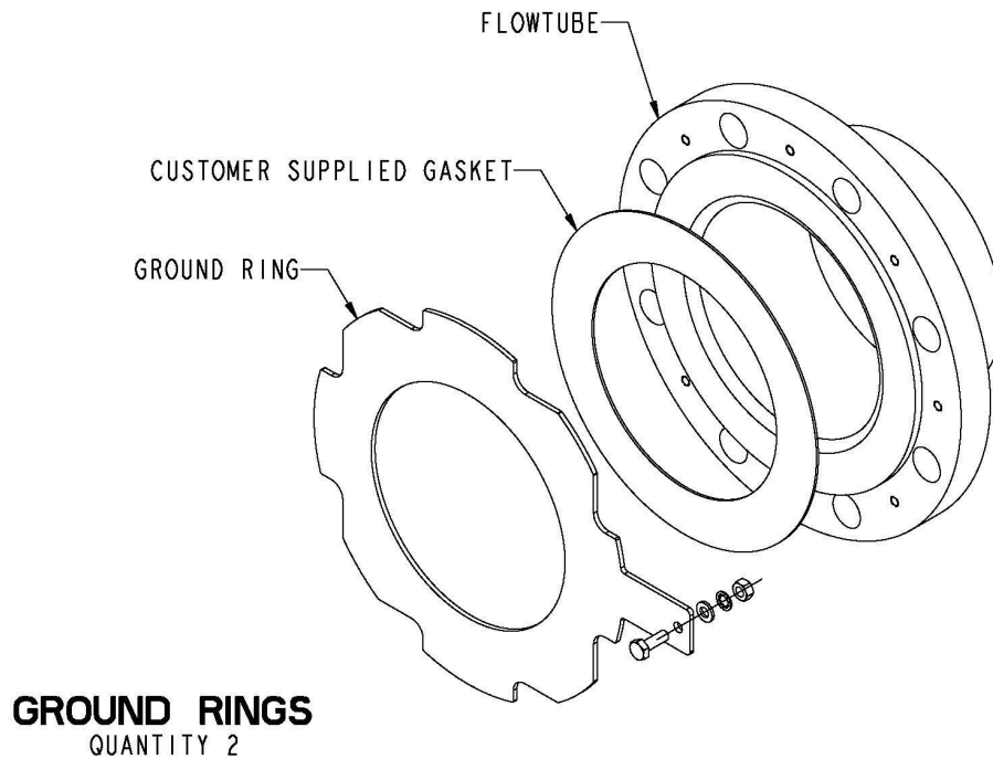
Abbildung 23: Messrohr 8705-M in Flanschbauweise 1/2 Zoll bis 36 Zoll (DN 15 mm bis 900 mm) Erdungsringe (P ≤ Class 900)
