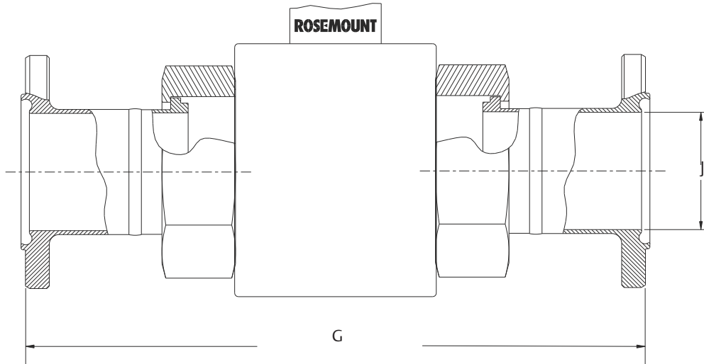
Abbildung 32: Messrohr 8721 in Hygienebauweise SMS1145
