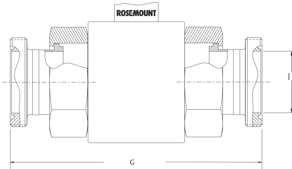
Abbildung 32: Messrohr 8721 in Hygienebauweise SMS1145
