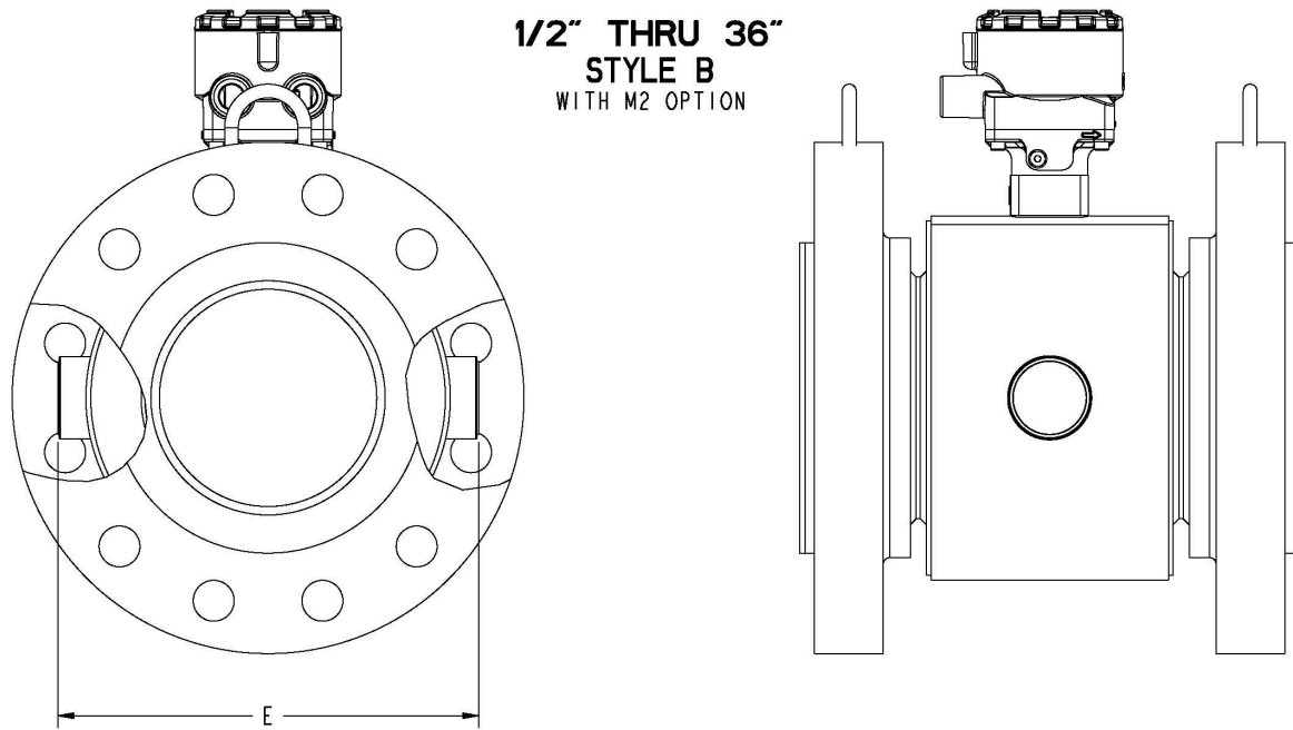
Abbildung 21: Messrohr 8705-M in Flanschbauweise 1/2 Zoll bis 36 Zoll (DN 15 mm bis 900 mm) M2/M4-Spulengehäuse (P ≤ Class 2500)
