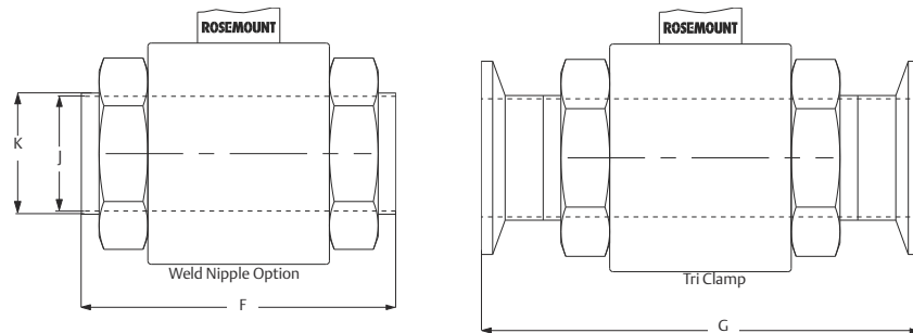
Abbildung 27: Messrohr 8721 in Hygienebauweise – Schweißnippel und Tri-Clamp
