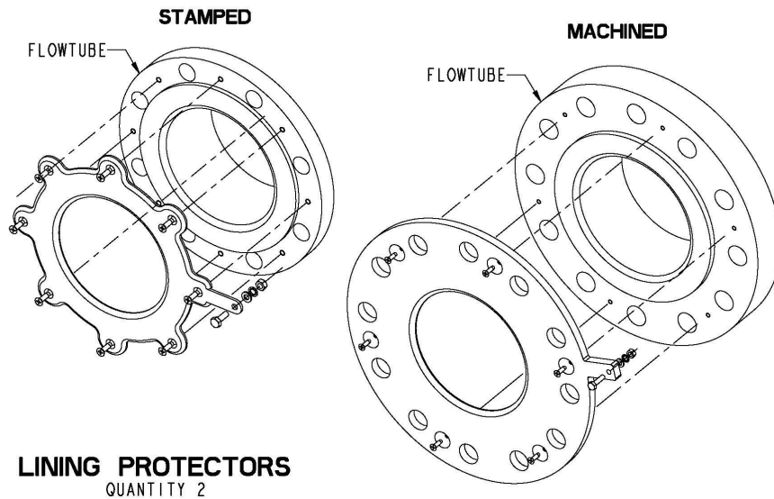
Abbildung 22: Messrohr 8705-M in Flanschbauweise 1/2 Zoll bis 36 Zoll (DN 15 mm bis 900 mm) Auskleidungsschutz (P ≤ Class 900)
