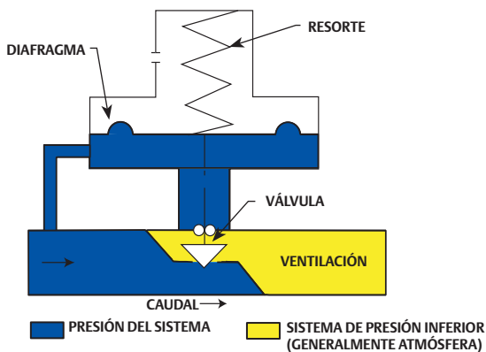
Figura 3. Válvula de alivio de acción directa
