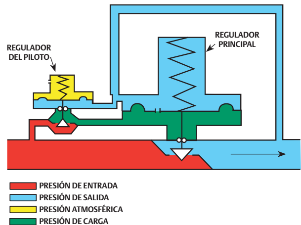
Figura 2. Regulador pilotado
