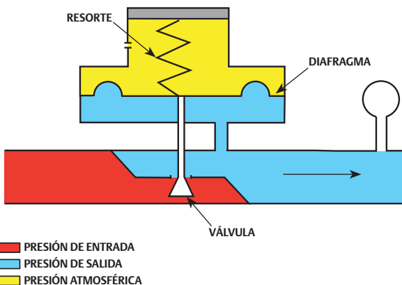
Figura 1. Reguladores de acción directa
