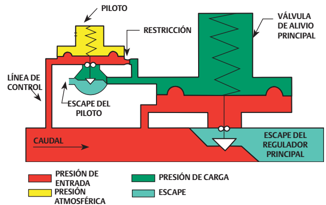
Figura 4. Válvula de alivio pilotada
