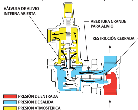
Figura 5. Alivio interno
