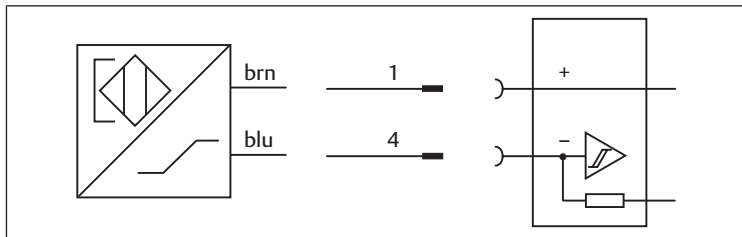
Abb. 1: Anschlussbild Sensor
