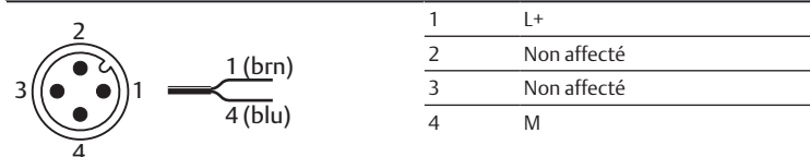
Fig. 1: Schéma de raccordement du capteur
