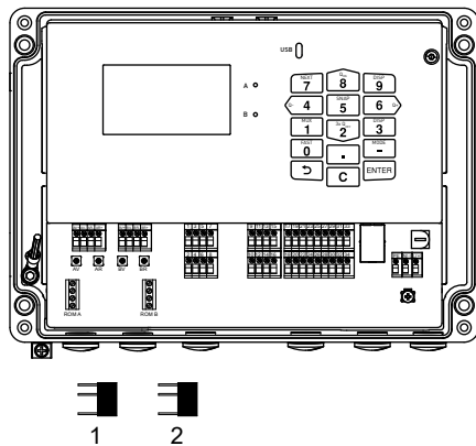
Fig. 7.11 : Mémoire SENSPROM
