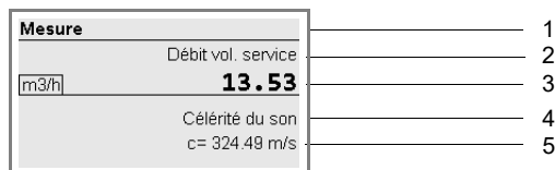
Fig. 9.4 : Affichage des valeurs mesurées
