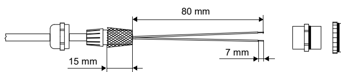
Fig. 7.30 : Câble préparé
