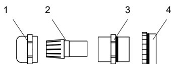
Fig. 7.29 : Presse-étoupe
