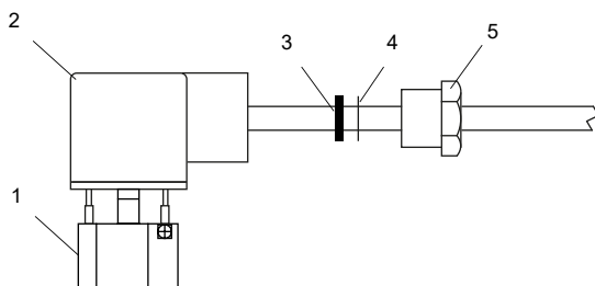
Fig. 7.25 : Montage du connecteur et du câble
