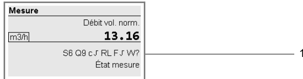
Fig. 9.5 : Affichage de la ligne d'état
