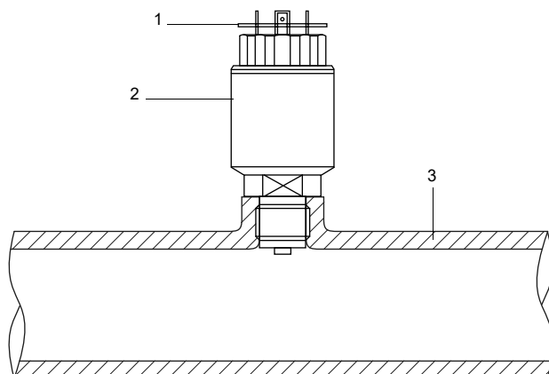
Fig. 6.75 : Transmetteur de pression monté
