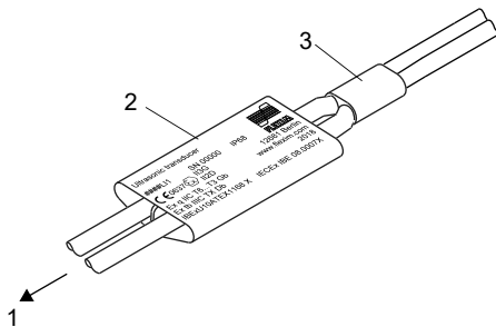
Fig. 6.17 : Plaquette signalétique au câble de capteurs
