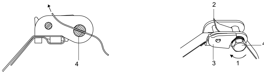
Fig. 6.29 : Fermeur à cliquet avec bande de serrage
