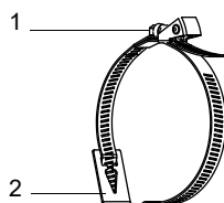
1 – vis du fermoir 2 – ressort métallique
