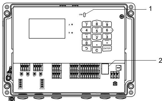
Fig. 7.31 : Interfaces de service au transmetteur
