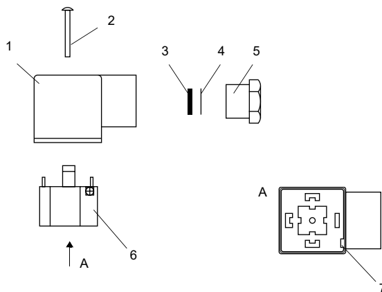
Fig. 7.21 : Connecteur démonté
