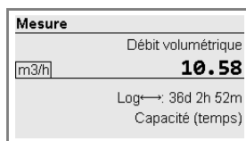
Fig. 9.9 : Informations sur la mémoire de valeurs mesurées
