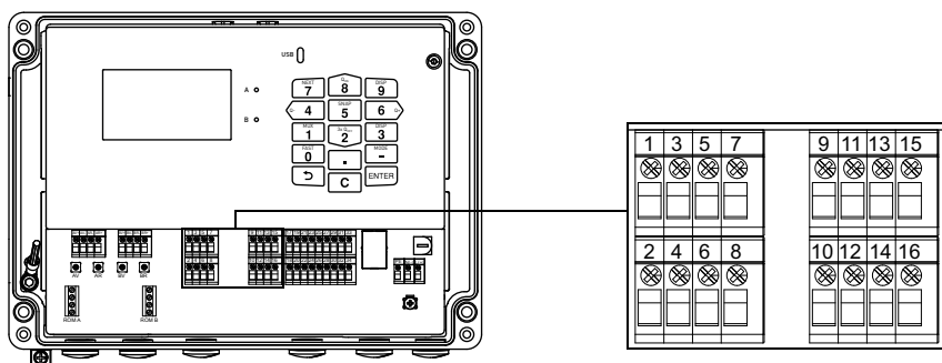
Fig. 7.28 : Raccordement des entrées au transmetteur
