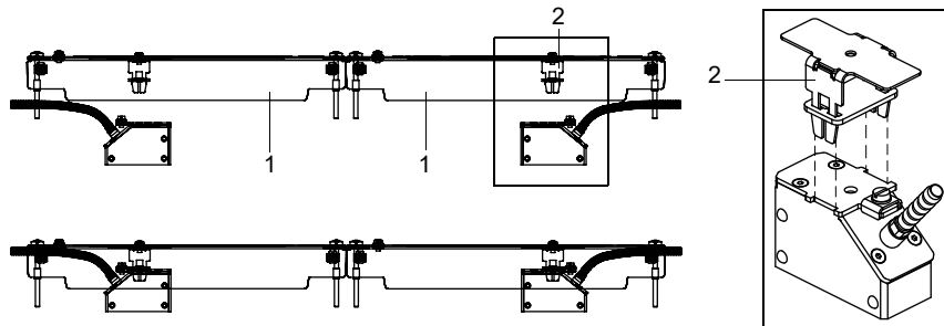
Fig. 6.38 : Montage des capteurs dans les caches
