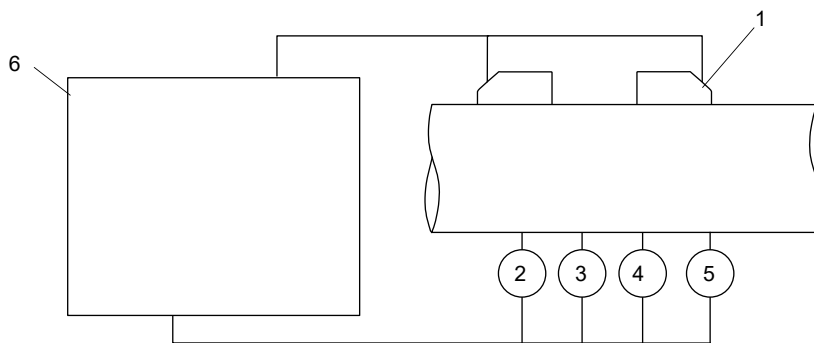
Fig. 20.1 : Détermination du débit d'énergie de gaz lors de la mesure du débit
