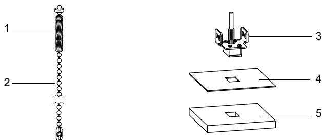
Fig. 6.71 : Sonde de température
