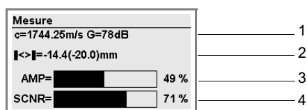
Fig. 9.1 : Écran de diagnostic
