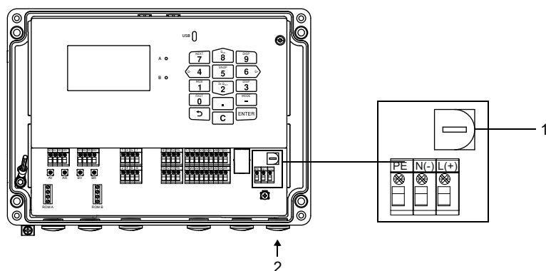
Fig. 7.13 : Raccordement de l'alimentation en tension au transmetteur
