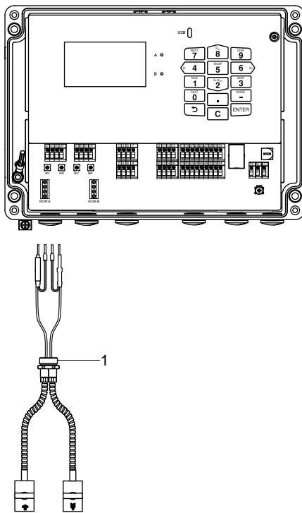
Fig. 7.4 : Raccordement du câble de capteurs avec gaine en acier inoxydable et extrémités dénudées au transmetteur
