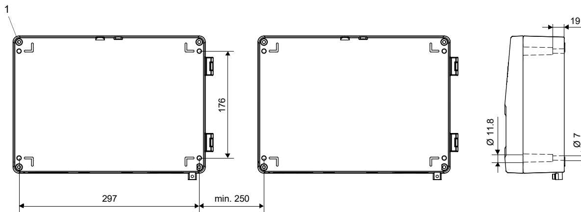
Fig. 6.4 : Transmetteur (dimensions en mm)
