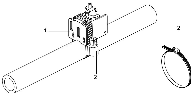
Fig. 6.59 : Capteur dans sa coquille de montage, monté à l'aide d'une bande de serrage avec fermoir
