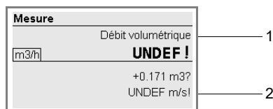
Fig. 13.1 : Vitesse d'écoulement en-dehors de la plage de validité
