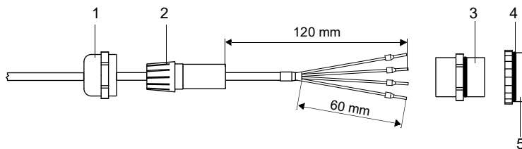
Fig. 7.18 : Préparation de la sonde de température
