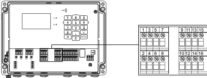
Fig. 7.17 : Raccordement des sondes de température au transmetteur
