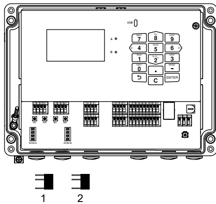
Fig. 7.11 : Mémoire SENSPROM
