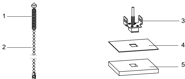
Fig. 6.64 : Sonde de température
