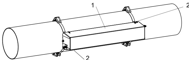
Fig. 6.57 : Variofix C avec capteurs sur la conduite
