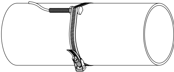
Fig. 6.61 : Sonde de température sur la conduite
