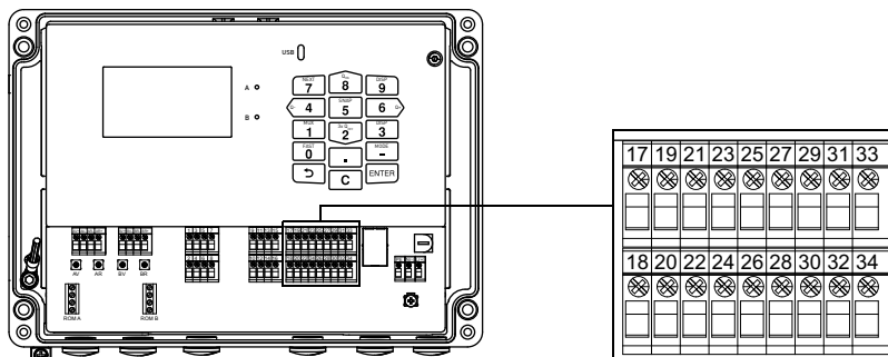
Fig. 7.15 : Raccordement des sorties au transmetteur
