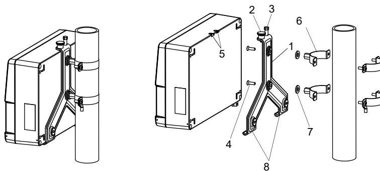
Fig. 6.6 : Vue de montage
