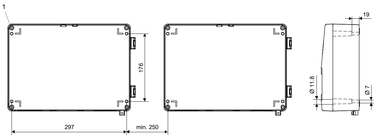
Fig. 6.4 : Transmetteur (dimensions en mm)
