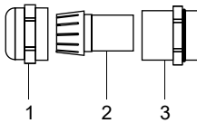
Fig. 7.14 : Presse-étoupe pour boîtier en aluminium
