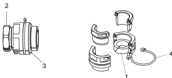
Fig. 7.22 : Presse-étoupe divisible
