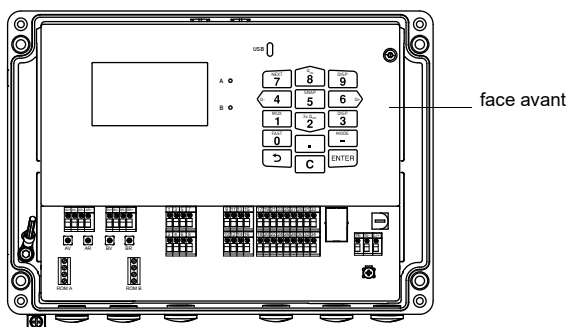
Fig. 2.1 : Transmetteur
