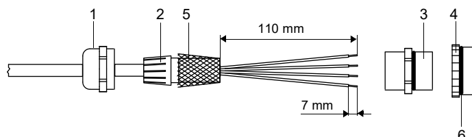
Fig. 7.19 : Préparation de la rallonge
