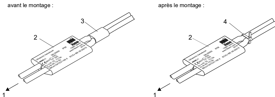
Fig. 6.9 : Plaquette signalétique au câble de capteurs
