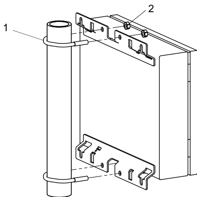
Fig. 6.5 : Vue de montage
