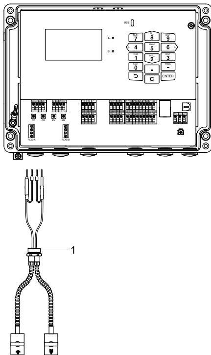
Fig. 7.4 : Raccordement du câble de capteurs avec gaine en acier inoxydable et extrémités dénudées au transmetteur
