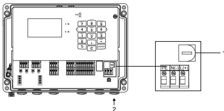
Fig. 7.13 : Raccordement de l'alimentation en tension au transmetteur
