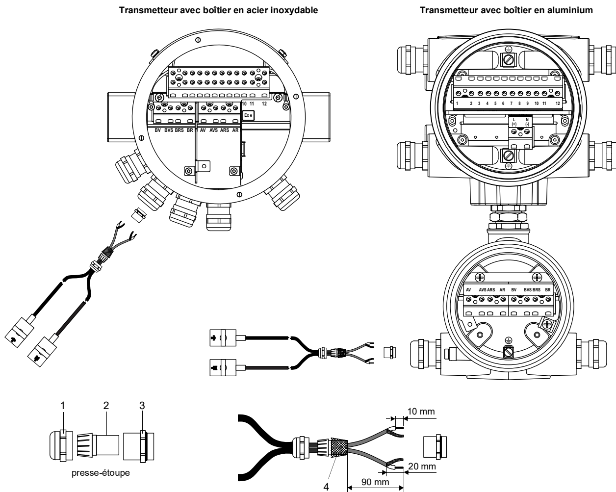
Fig. 7.5 : Raccordement du câble de capteurs avec gaine plastique et extrémités dénudées au transmetteur
