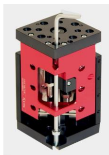
Fig. 8 Modules de course à visser
