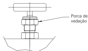
Orifício H1-3/8" e 5/8", H5 Tipos de junta de vedação PTFE e com grafite
