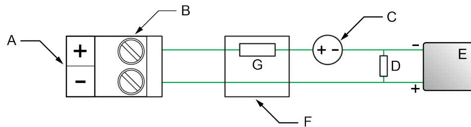
Figura 4-9: Cableado de salida de mA en una área clasificada
