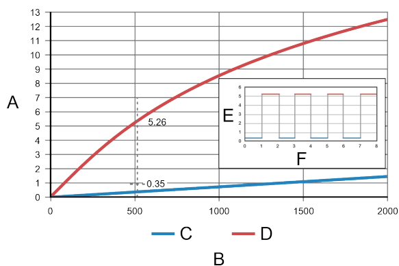
Figura 4-8: Alimentación de 24 V CC
