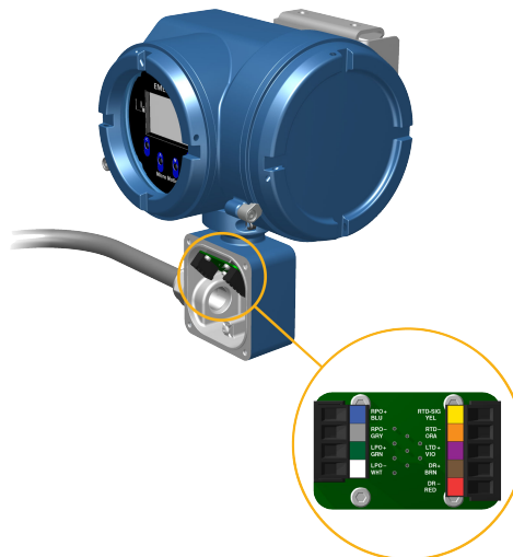
Figura 3-11: Conexiones de cableado de transmisor a sensor de nueve hilos
