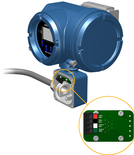
Figura 3-10: Conexiones de cableado de transmisor a sensor de cuatro hilos
