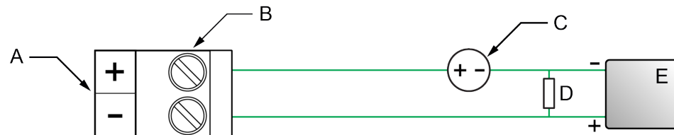
Figura 4-6: Cableado FO y DO para conectar a un sistema de medición
