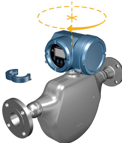
Figura 3-13: Rotación del cabezal del transmisor
