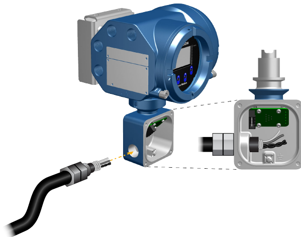
Figura 3-9: Paso de cables del sensor
