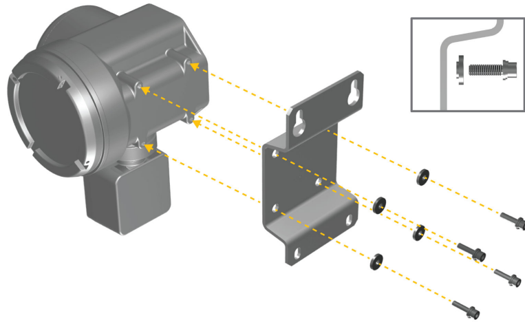
Figura 3-2: Soporte de montaje a transmisor de acero inoxidable
