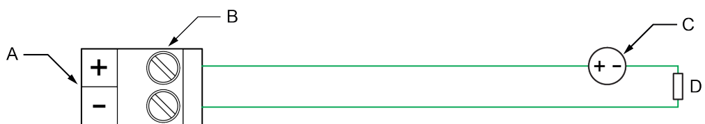
Figura 4-7: Cableado de DO con un relé o indicador
