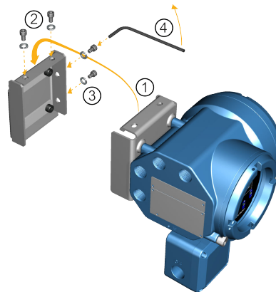
Figura 3-5: Montaje y fijación de un transmisor de aluminio al soporte de montaje
