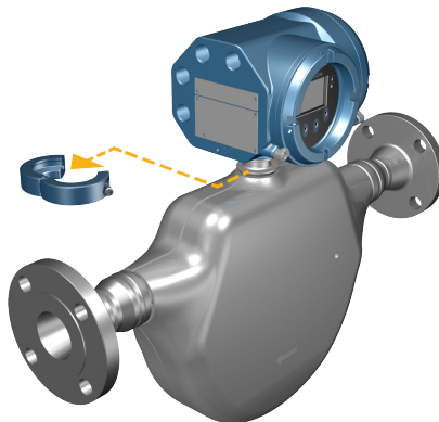
Figura 3-12: Extracción de la abrazadera del sensor
