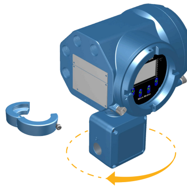
Figura 3-17: Rotación de la caja de conexiones debajo del transmisor
