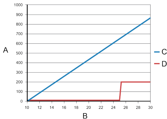
Figura 4-5: Salida de mA: Resistencia de lazo
