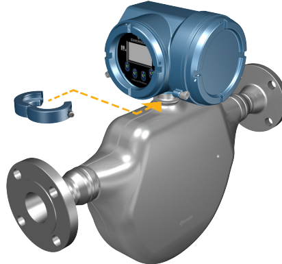
Figura 3-14: Volver a fijar la abrazadera del sensor
