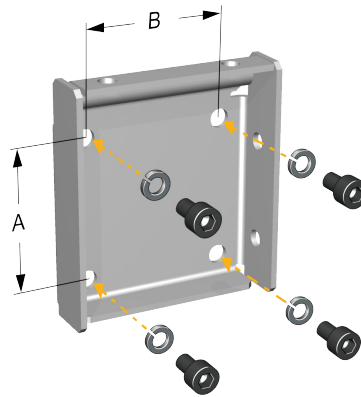
Figura 3-3: Soporte de montaje en pared y dimensiones para un transmisor de aluminio
