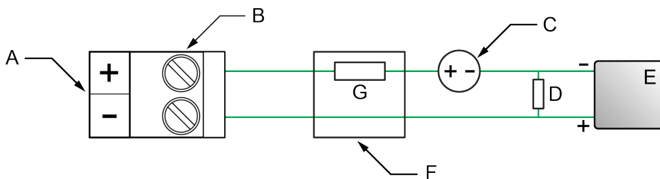
Figura 4-11: Cableado clasificado FO y DO
