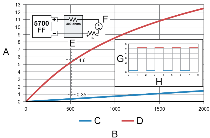
Figura 4-12: Alimentación de 24 V CC con una barrera de 300 Ω
