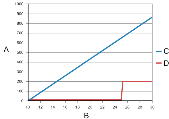
Figura 4-10: Salida de mA: Resistencia de lazo
