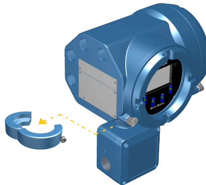
Figura 3-16: Extracción de la abrazadera
