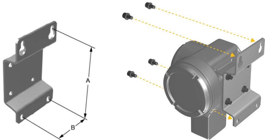
Figura 3-4: Soporte de montaje en pared y dimensiones para un transmisor de acero inoxidable
