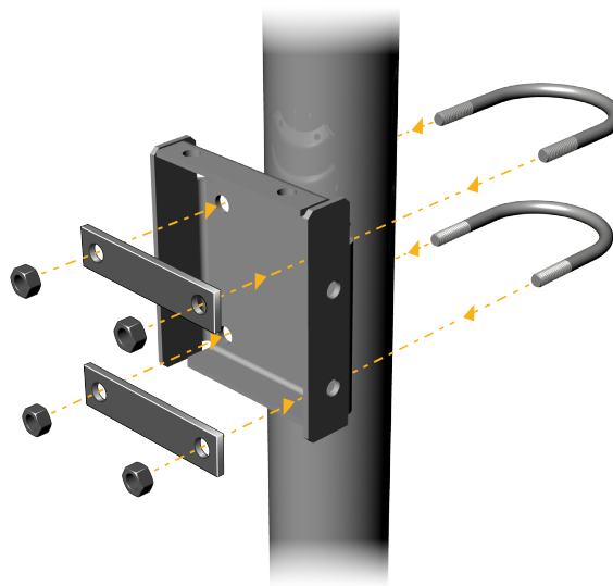
Figura 3-6: Fijación de soporte de montaje en poste para un transmisor de aluminio
