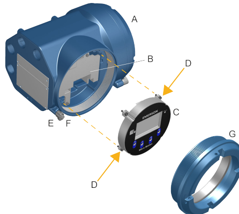
Figura 3-15: Componentes del indicador
