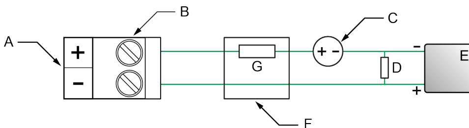
Figura 4-11: Fiação classificada da SF e da SD
