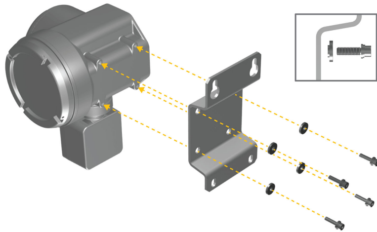
Figura 3-2: Montar o suporte a um transmissor de aço inoxidável
