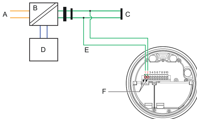
Figura 4-3: Cabeamento para PROFIBUS-PA 5700
