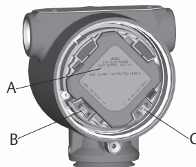
Abbildung 3-1: Konfiguration des Schalters und der Steckbrücke des Messumformers (Plantweb)
