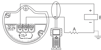
Abbildung 4-1: Messumformerverkabelung (Plantweb Gehäuse)
