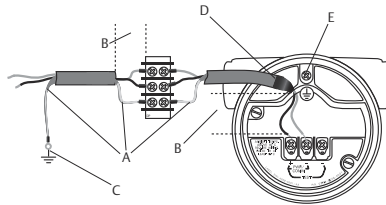
Abbildung 4-3: Verkabelung
