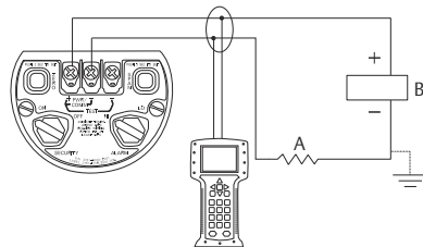
Abbildung 4-2: Messumformerverkabelung (Anschlusskasten-Gehäuse)
