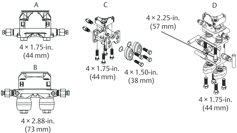
Abbildung 1-1: Gebräuchliche Messumformer-Baugruppen
