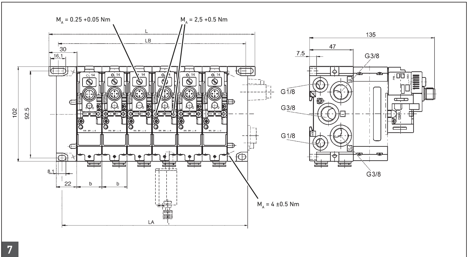
Maßzeichnung CD01-PA mit M12-Anschluss / CD01-PA dimensional drawing with M12 connector / Dessin coté CD01-PA avec raccord M12 / Disegno quotato CD01-PA con attacco M12 / Esquema acotado del CD01-PA con conexión M12 / Måttitning CD01-PA med M12-anlutning
