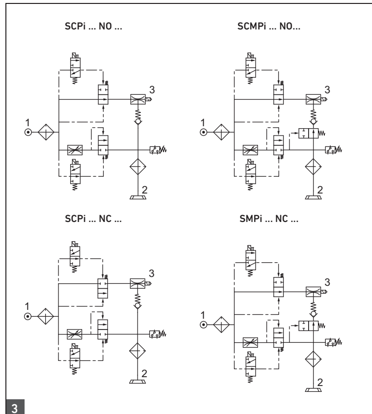
Pneumatikschaltpläne
