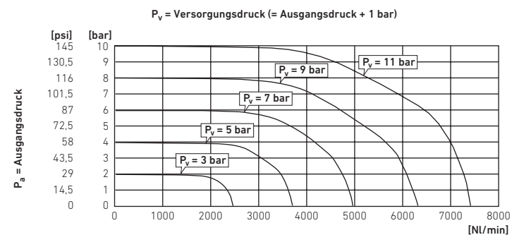
Durchflusskennlinien des EV12-Druckregelventils Typ C
