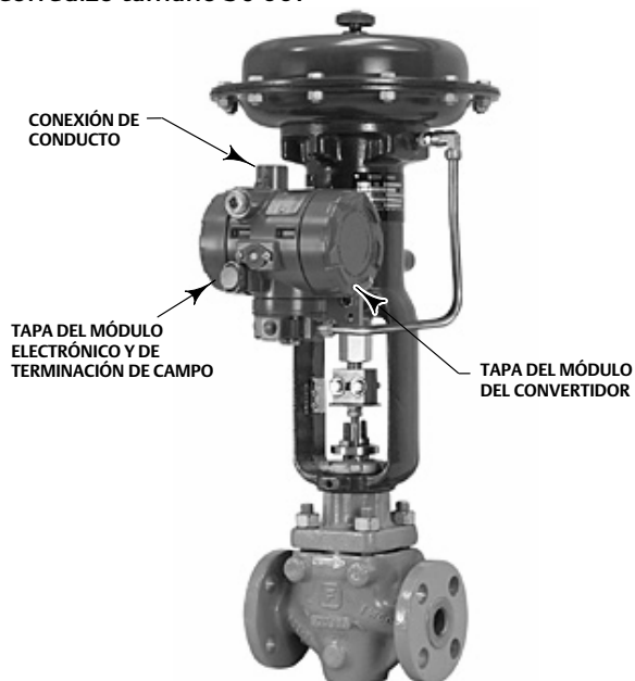
Figura 3. Transductor electroneumático Fisher i2P-100 montado sobre un actuador de vástago corredizo tamaño 30 667
