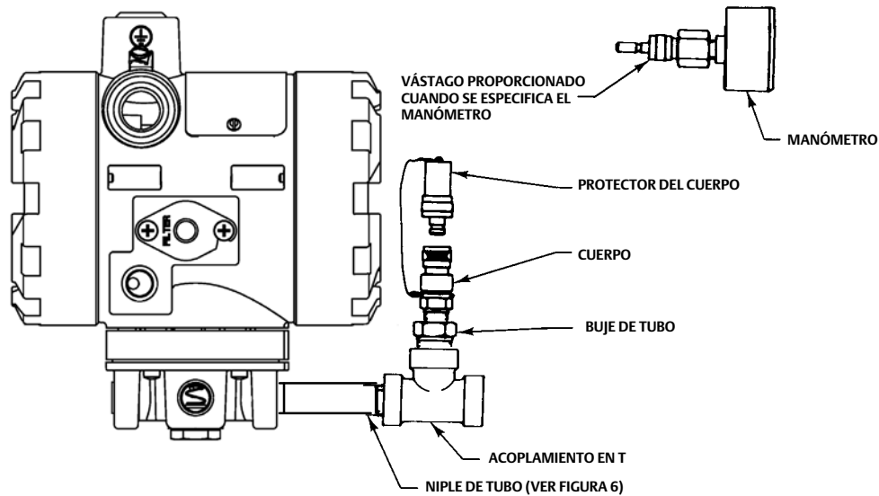
Figura 7. Acoplamiento de diagnóstico para el Transductor Fisher i2P-100
