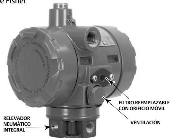
Figura 1. Transductor electroneumático i2P-100 de Fisher
