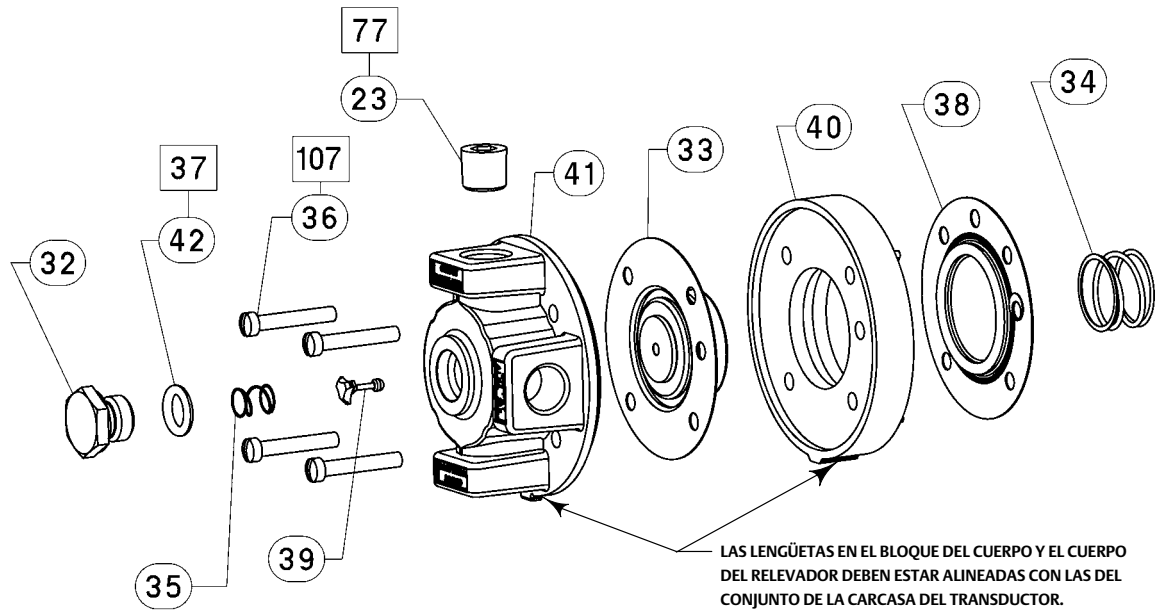
Figura 14. Conjunto de relevador Fisher i2P-100
