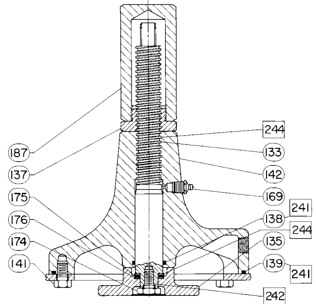
Figura 19. Batentes de deslocamento ajustáveis para cima para atuadores de tamanhos 70/70i e 87 (Estilo 1)
