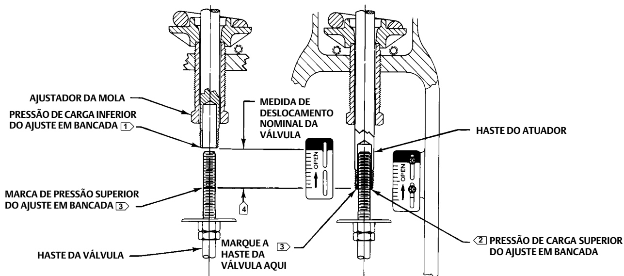
Figura 4. Ajuste do ajuste em bancada
