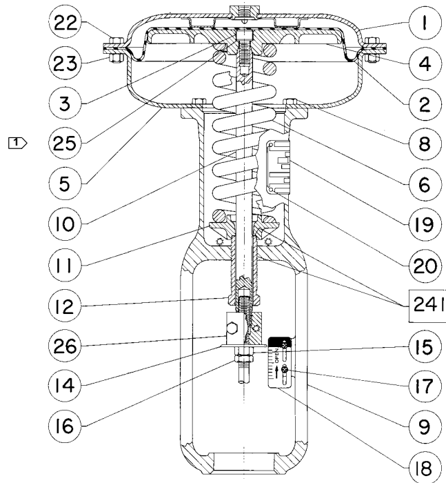
Figura 6. Atuador Fisher 657 tamanhos 30 a 60
