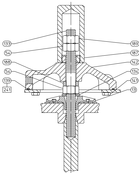
Figura 20. Batente de deslocamento ajustável para baixo montado na caixa para atuadores de tamanhos 30/30i e 40/40i (Estilo 2)
