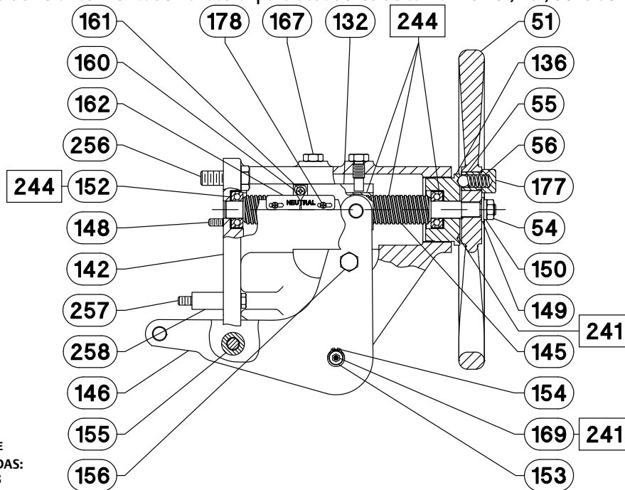
Figura 16. Conjunto de volante montado na lateral para atuadores de tamanho 45i, 46i, 50i e 60i
