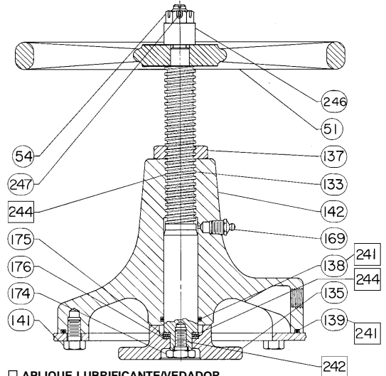
Figura 12. Conjunto de volante montado no topo para atuadores tamanhos 70/70i a 87
