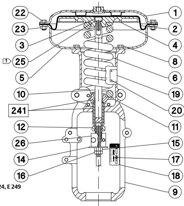
Figura 7. Atuador Fisher 657 Tamanho 30i a 60i
