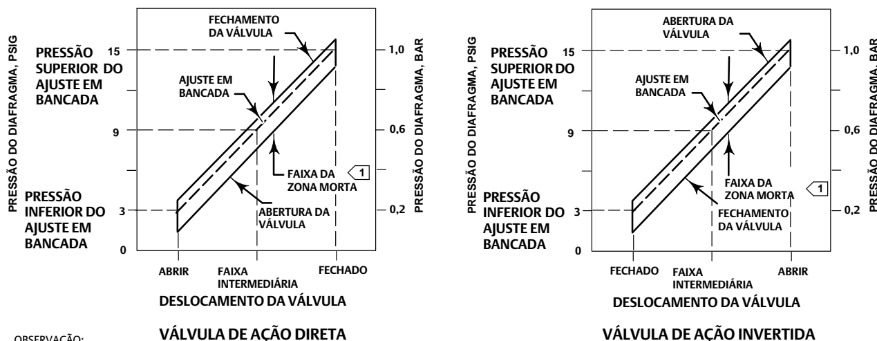
Figura 5. Resposta típica da válvula à zona morta
