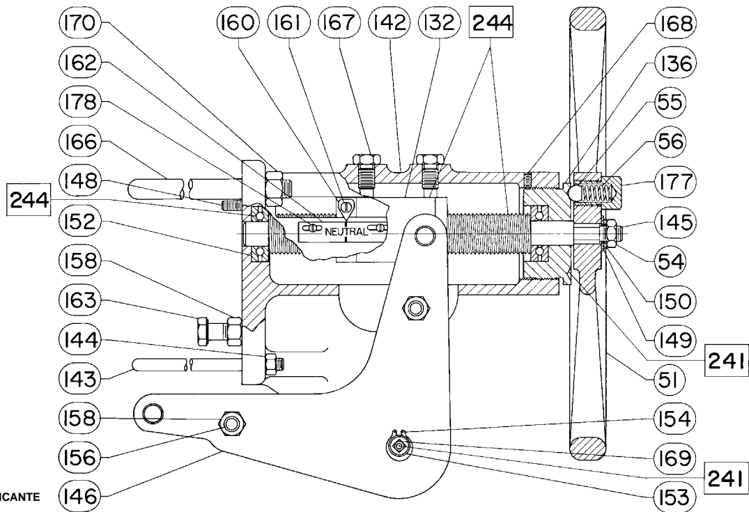
Figura 15. Conjunto de volante montado na lateral para atuadores de tamanhos 45, 46, 50 e 60
