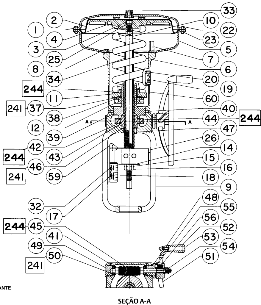
Figura 17. Atuadores Fisher 657 tamanhos 70 e 87 com volante montado na lateral
