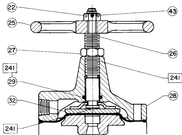
Figure 6. Volant supérieur, tailles 3A et 4A
