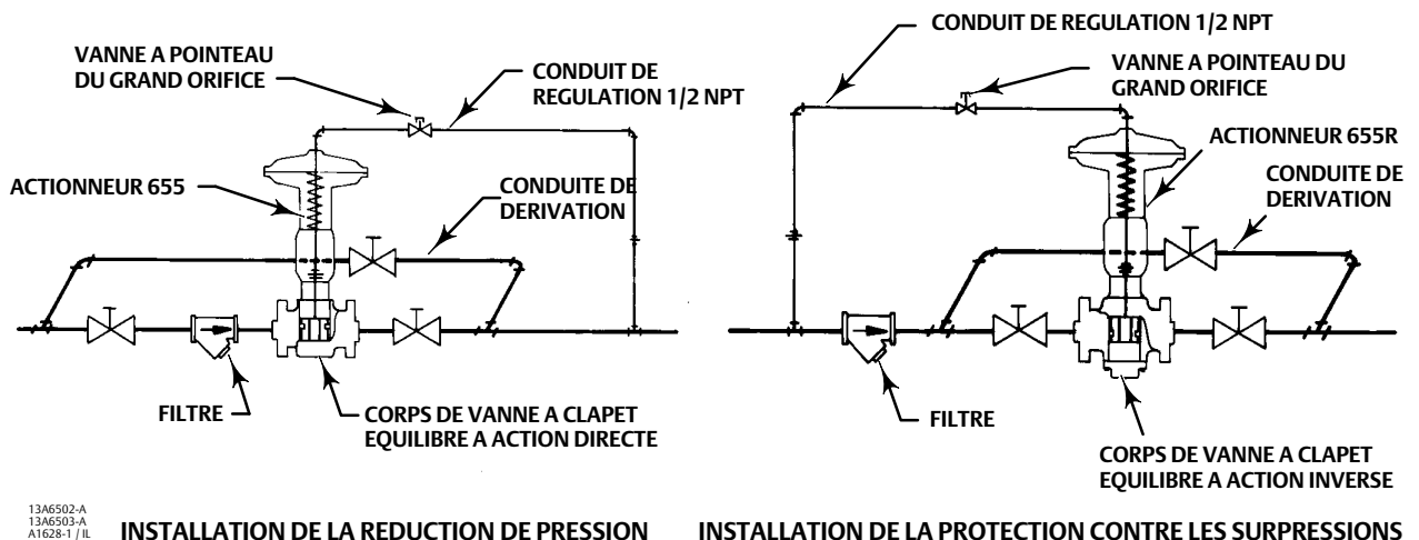
Figure 2. Schéma d'installation type
