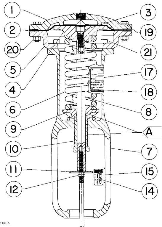
Figure 4. Actionneur Fisher 655
