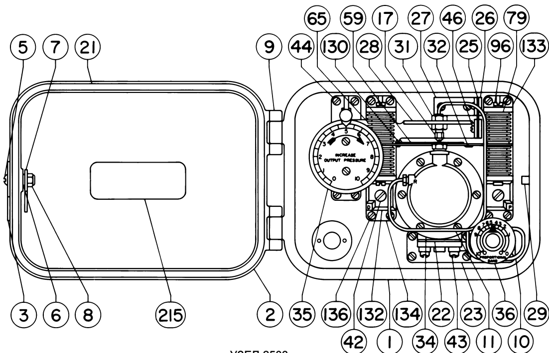
УЗЕЛ 2506
