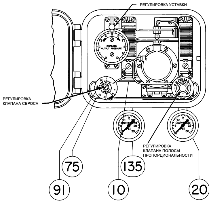
УЗЕЛ 2516
