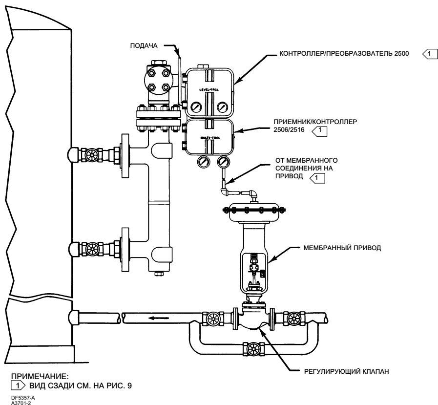
Рис. 10. Стандартная установка преобразователя с приемником и регулирующим клапаном в сборе
