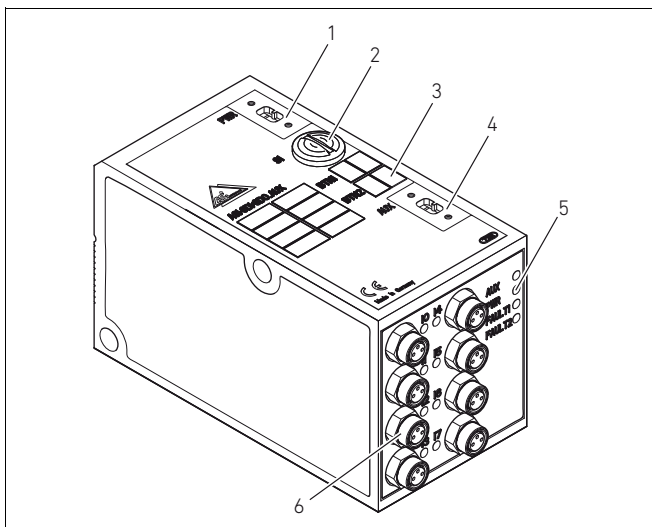
Fig. 2: Coupleur de bus, exemple 8DI/8DO-AUX
