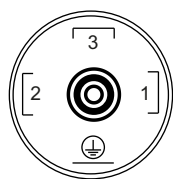
Fig. 7.27: Contactos machos del transmisor de presión
