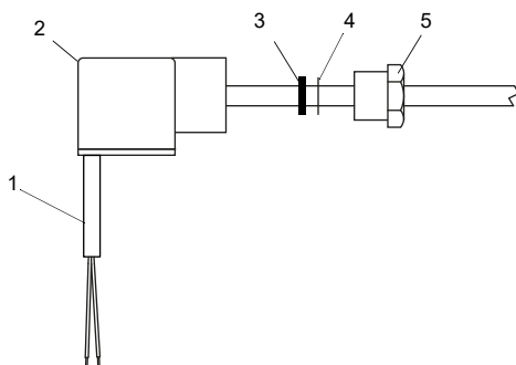
Fig. 7.22: Montaje del cable
