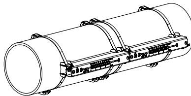
Fig. 6.19: Porta-transductor Variofix L (configuración en modo de reflexión)
