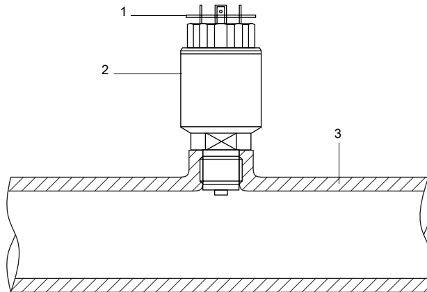
Fig. 6.75: Transmisor de presión montado
