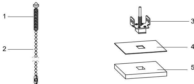
Fig. 6.71: Sensor de temperatura
