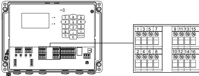
Fig. 7.16: Conexión de las entradas al transmisor
