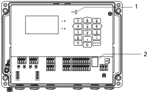
Fig. 7.31: Interfaces de servicio en el transmisor
