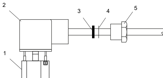
Fig. 7.25: Montaje del conector y del cable
