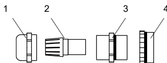
Fig. 7.29: Prensaestopas
