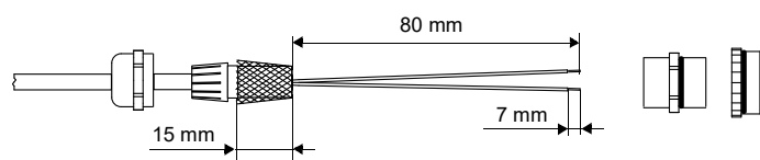
Fig. 7.30: Cable confeccionado
