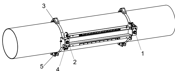
Fig. 6.57: Riel en la tubería
