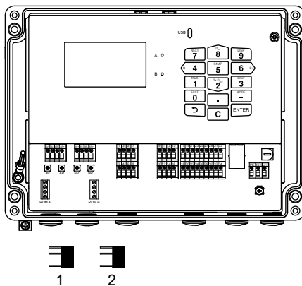
Fig. 7.11: Memoria SENSPROM
