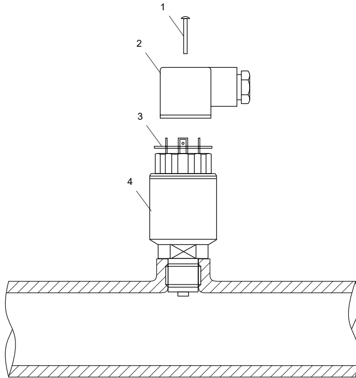
Fig. 7.26: Fijación del conector
