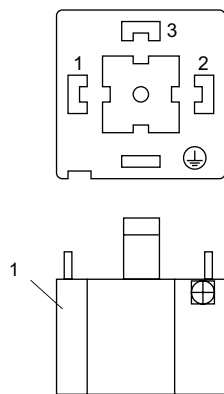
Fig. 7.24: Conexión de bornes (conector)
