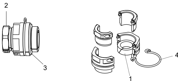
Fig. 7.32: Prensaestopas partido
