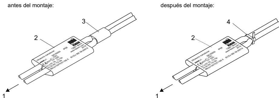
Fig. 6.9: Placa de características en el cable del transductor
