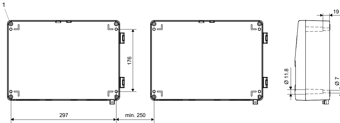
Fig. 6.4: Transmisor (dimensiones en mm)
