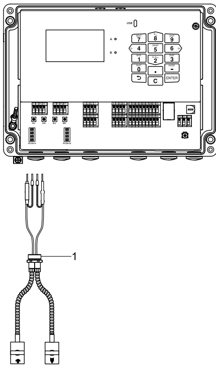
1 – prensaestopas
