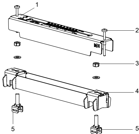
Fig. 6.12: Desmontaje del Variofix L
