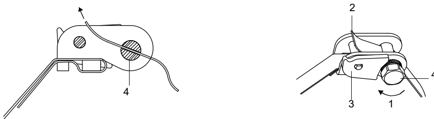
Fig. 6.53: Cierre de trinquete con cinta de sujeción
