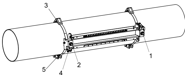
Fig. 6.49: Riel en la tubería
