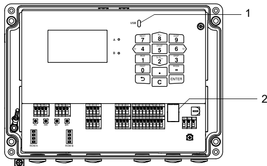
Fig. 7.17: Interfaces de servicio en el transmisor
