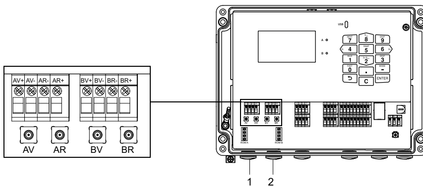
Fig. 7.1: Conexión de los transductores en el transmisor
