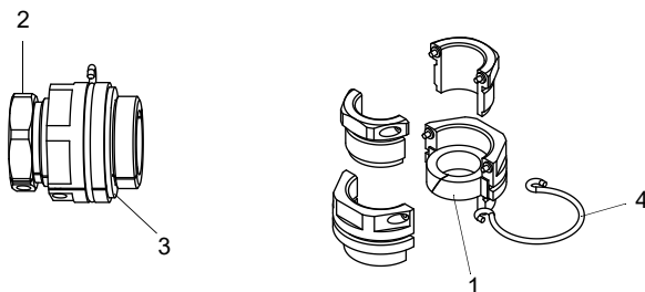
Fig. 7.18: Prensaestopas partido
