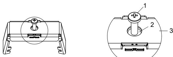
Fig. 6.55: Estribo elástico
