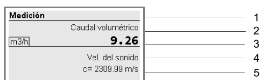
Fig. 9.2: Visualización de los valores de medición
