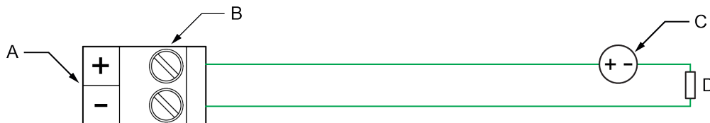
Рисунок 4-7. Подключение дискретного выхода к реле или индикатору
