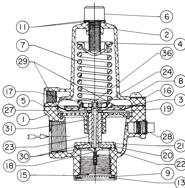
Figur 1. Type 289 samling
