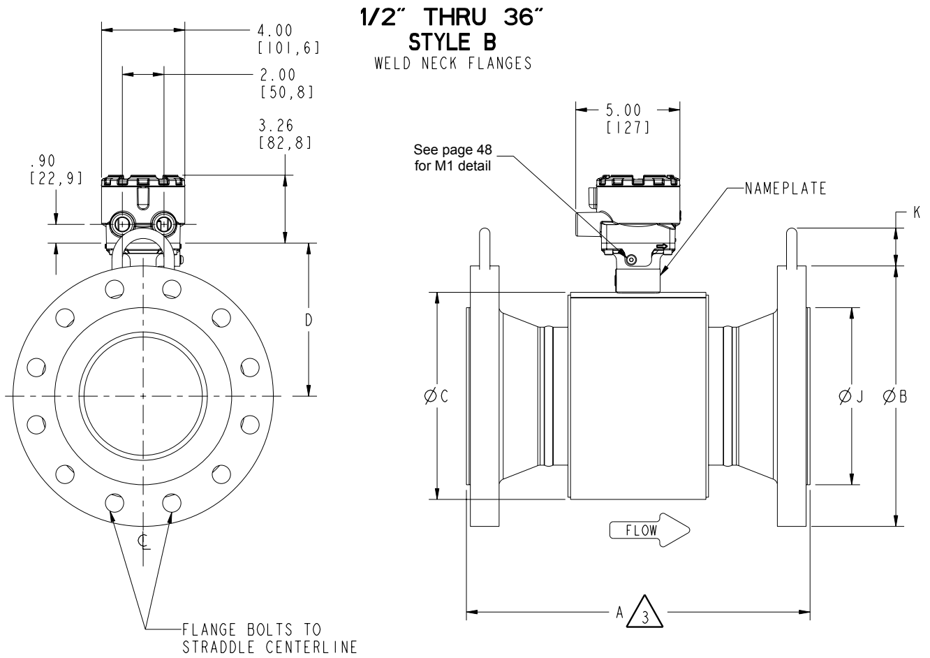
Figura 16: Sensor bridado 8705-M de 1/2 in a 36 in (DN de 15 mm a 900 mm) bridas con cuello soldadas - (P ≤ clase 600 reducida)
