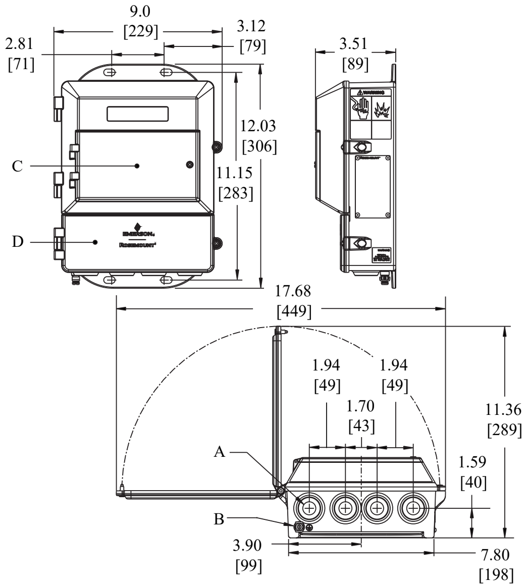
Figura 12: Dimensiones del transmisor de montaje en pared 8712
