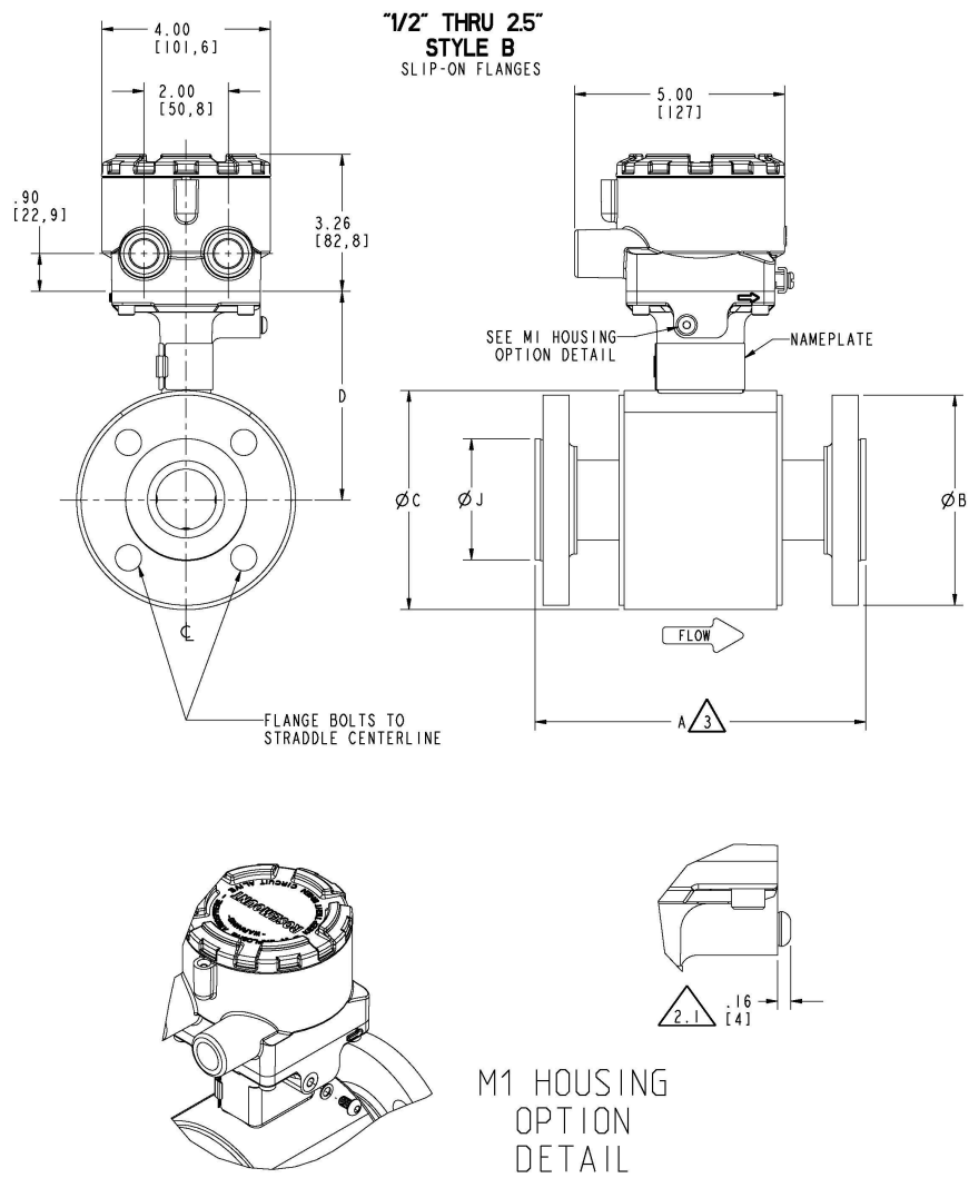
Figura 19: Sensor bridado 8705-M de 1/2 in a 24 in (DN de 15 mm a 600 mm), bridas deslizantes - alta presión (P ≤ clase 900)
