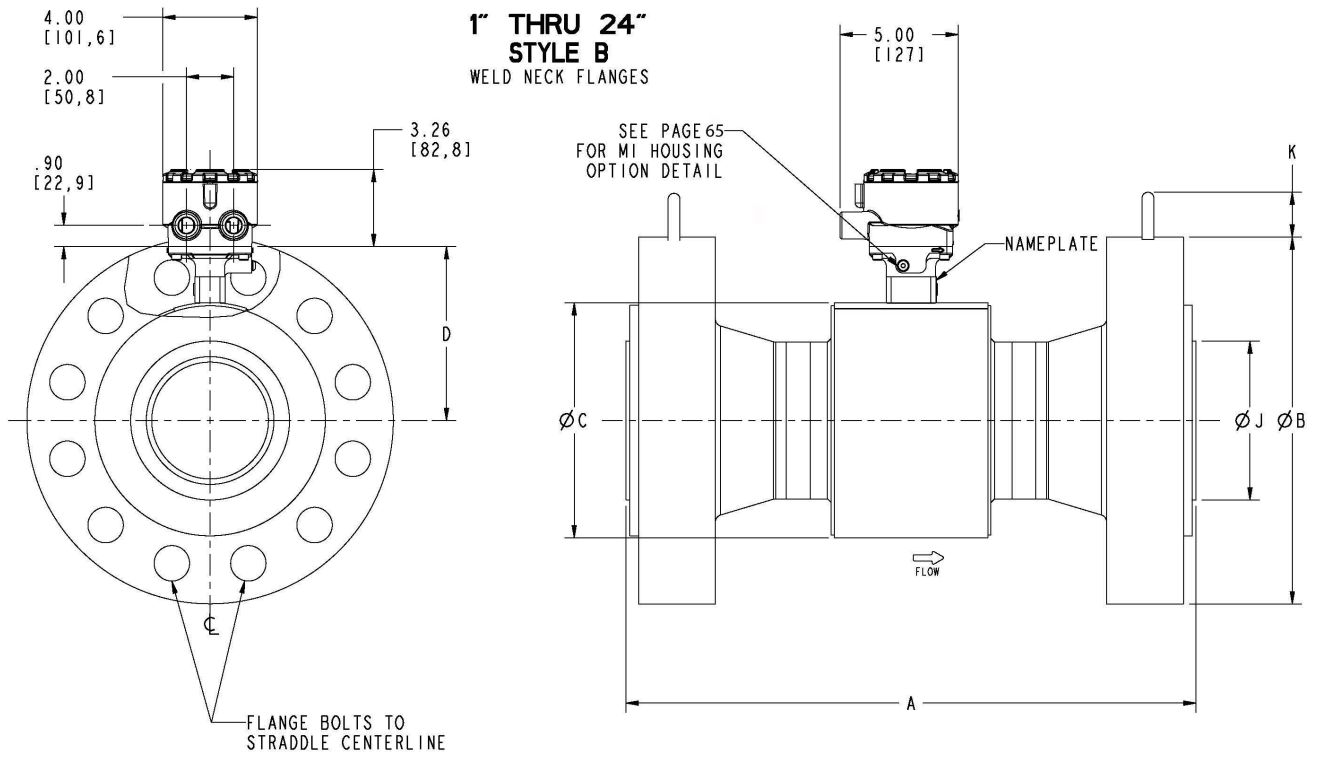
Figura 20: Sensor bridado 8705-M de 1 in a 24 in (DN de 25 mm a 600 mm) bridas con cuello soldadas - (P ≤ clase 2500)
