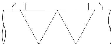
Afb. 3.5: Reflectieopstelling met 1 straal en 4 meetpaden
