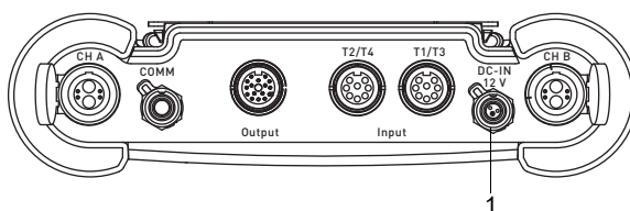
Afb. 7.3: Aansluiting van de netadapter op de transmitter
