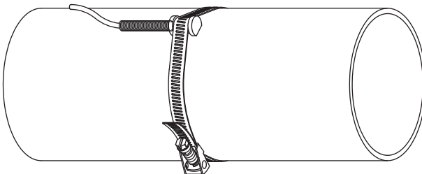
Afb. 6.17: Temperatuursensor op de buis
