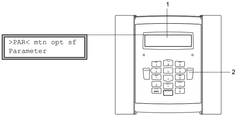
Afb. 4.2: Bedieningsveld van de transmitter
