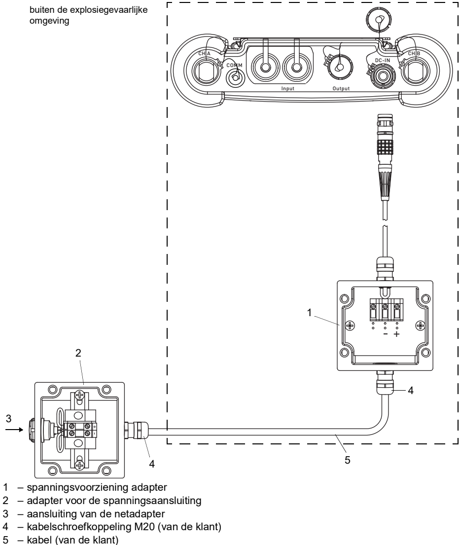
Afb. 7.20: De externe adapters aansluiten
