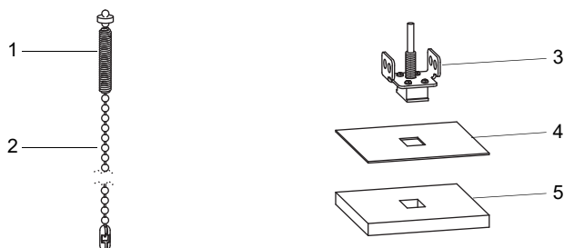
Afb. 6.20: Temperatuursensor
