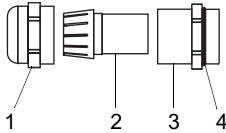
Afb. 7.24: Kabelschroefkoppeling
