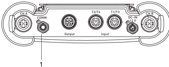
Afb. 7.12: Aansluiting van de service-interface op de transmitter
