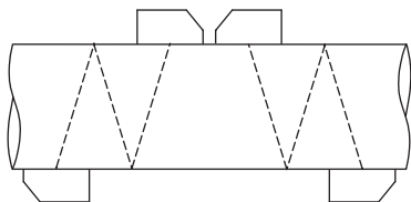
Afb. 3.4: Doorstralingsopstelling met 2 stralen en 3 meetpaden
