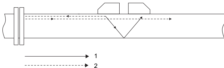
Afb. 3.10: Verspreiden de ultrasonische golven
