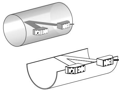
Afb. 3.7: 2 meetpaden op één niveau
