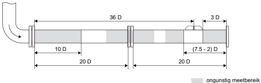
Afb. 3.12: Bereik voor het meetpunt met gunstig stromingsprofiel en geringe invloed van stoorgeluid
