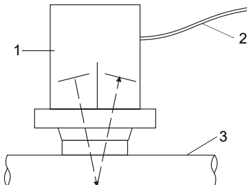
Afb. 20.1: Meetprincipe
