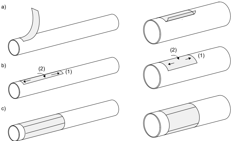
Afb. 6.10: De dempingsmatten bevestigen
