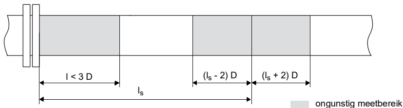
Afb. 3.11: Te voorkomen meetpunten
