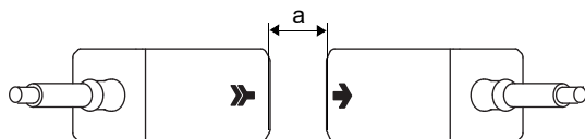
Afb. 6.13: De sensoren en de sensorafstand afstellen
