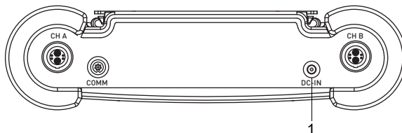
Afb. 7.19: Aansluiting van de netadapter op de transmitter FLUXUS *608**-F2
