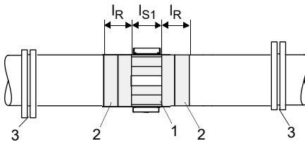
Afb. 6.12: Buisbuitendiameter > 900 mm
