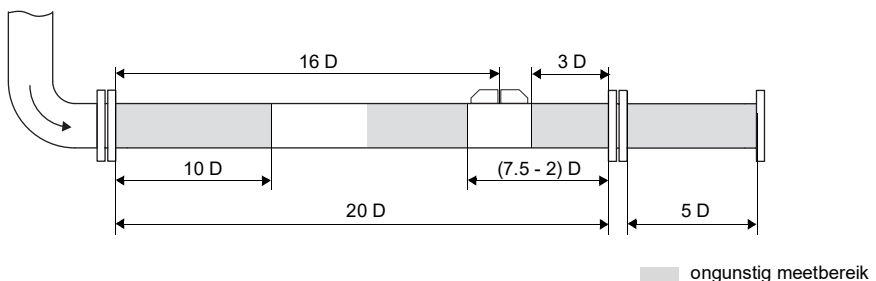
Afb. 3.13: Bereik voor het meetpunt met geringe invloed van stoorgeluid en niet volledig gevormd stromingsprofiel
