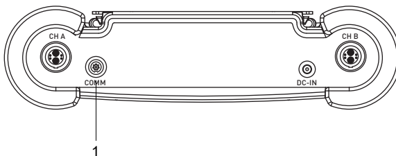
Afb. 7.30: Aansluiting van de service-interface op de transmitter FLUXUS *608**-F2
