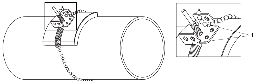
Afb. 6.21: Temperatuursensor op de buis
