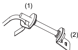
Afb. 6.18: FLEXIM-spanslot
