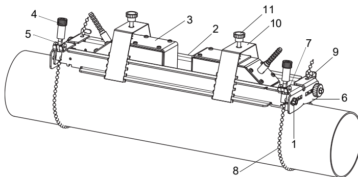
Afb. 6.15: Variofix-rail met kettingen
