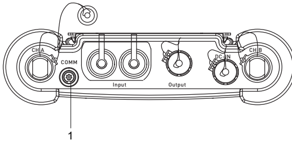
Afb. 7.29: Aansluiting van de service-interface op de transmitter FLUXUS *608**-A2
