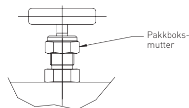
H1- \frac{3}{8} " OG \frac{5}{8} " ÅPNING, H5 PTFE og grafitt pakkbokstyper
