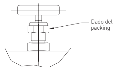
TIPO H1 CON ORIFIZIO DA 3/8" E 5/8", H5, con packing in PTFE e grafite
