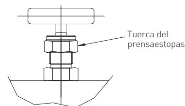
TIPOS H1 DE PASO 3/8" Y 1/2", H5 Empaquetaduras P.T.F.E. y grafito
