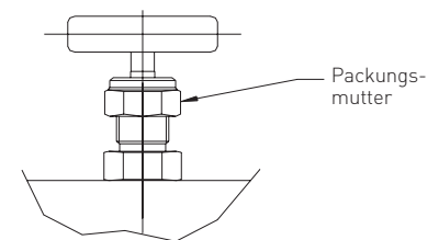
TYPEN H1-3/8" UND 1/2" ÖFFNUNG, H5 PTFE + Graphitpackung
