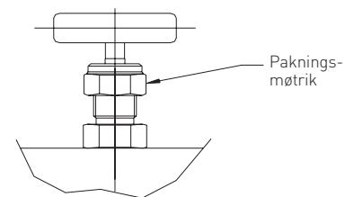
H1- \frac{3}{8} " OG \frac{1}{2} " ÅBNING, H5 PTFE og Graphite pakningstyper
