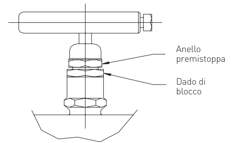
TIPO H7/H1-2, H7, SERIE A
