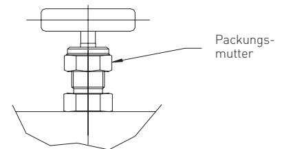
TYPEN H1-3/8" UND 1/2" ÖFFNUNG, H5 PTFE + Graphitpackung
