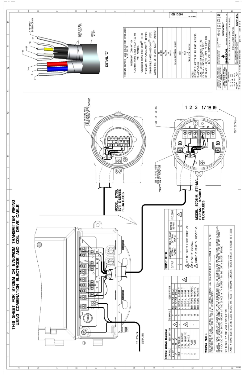
Figura 5-7: Cablaggio con multicavo
