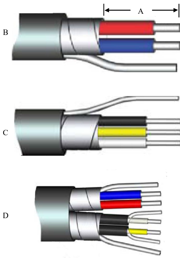
Figura 5-4: Estremità dei cavi
