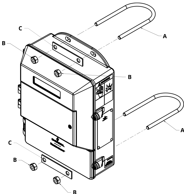
Figura 4-1: Staffa di montaggio
