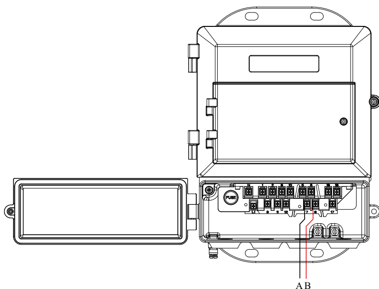
Figura 5-12: Cablaggio dell'uscita analogica
