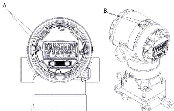
Figura 3-6: Botões Internos e Externos da LOI
