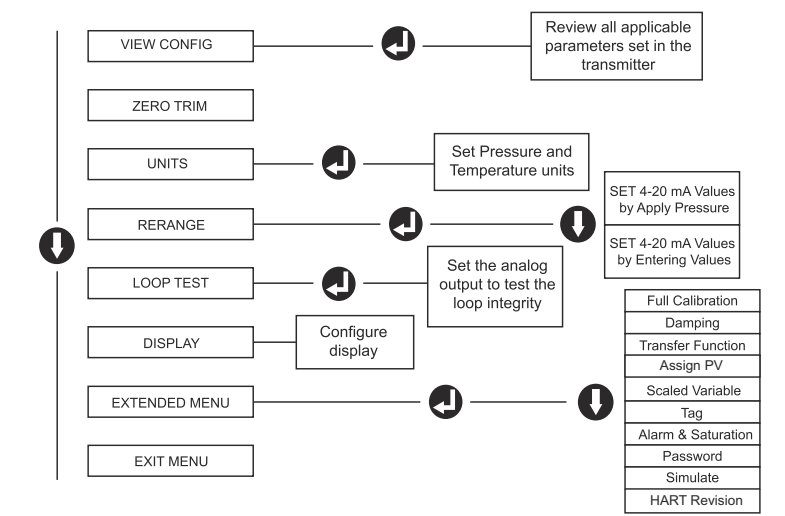
Figura 3-7: Menu da LOI
