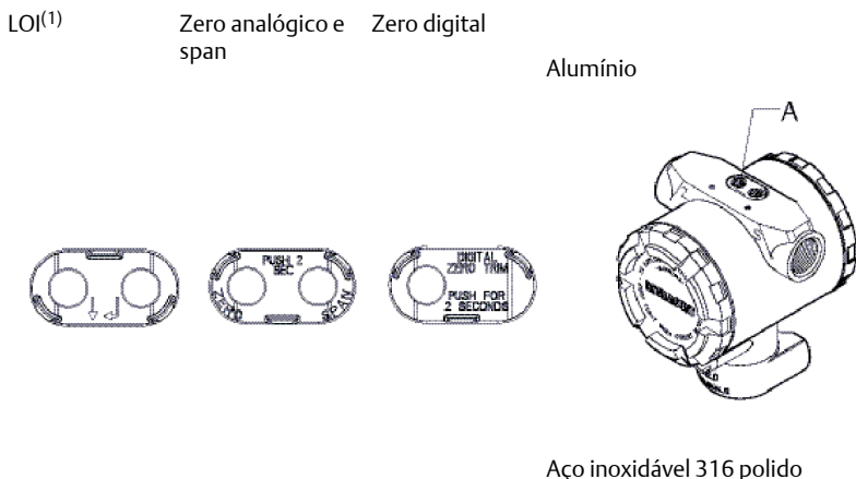
Figura 3-8: Botões de Configuração Externos ou no Lado Traseiro/dos Terminais
