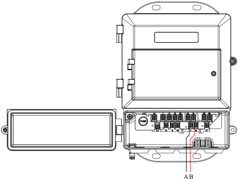
Figura 5-12: Cableado de la salida analógica
