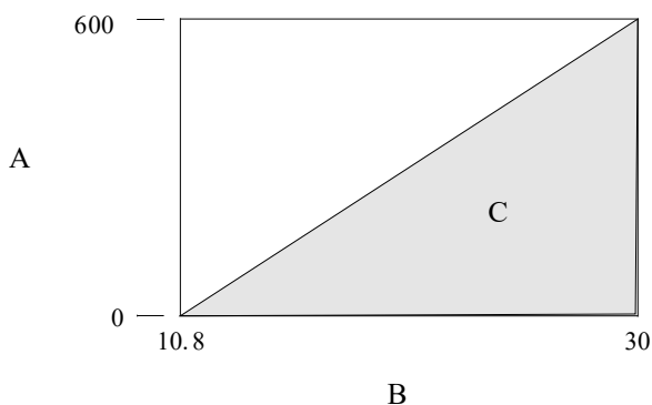
Figura 5-13: Limitaciones de carga del lazo analógico
