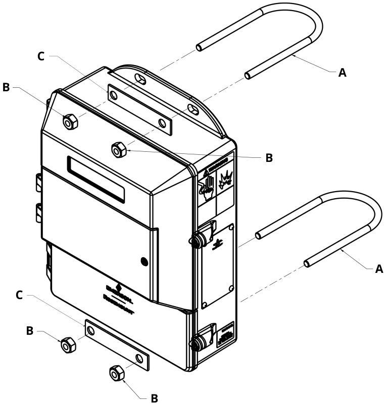
Figura 4-1: Soporte de montaje
