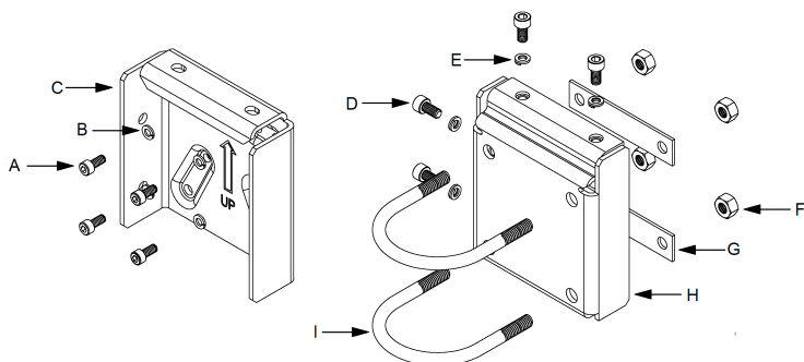
Figura 4-3: Componentes del juego de soporte de montaje
