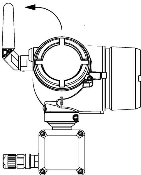
Figura 2-1: Posición de la antena
