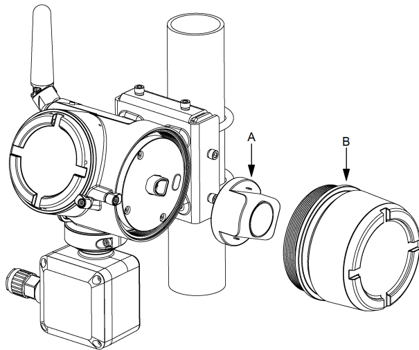
Figura 4-8: Instalación del módulo de alimentación
