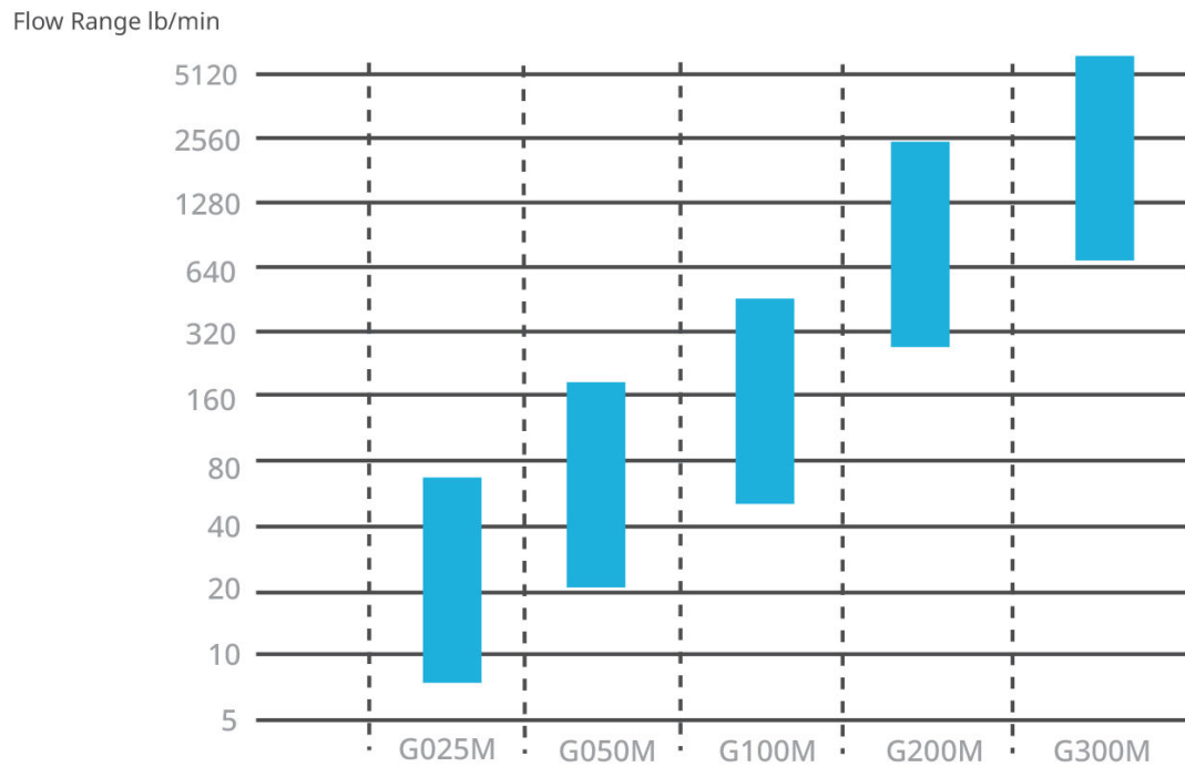
Figura 2: Faixa da medição de vazão e especificações de desempenho da Série G: sistema imperial
