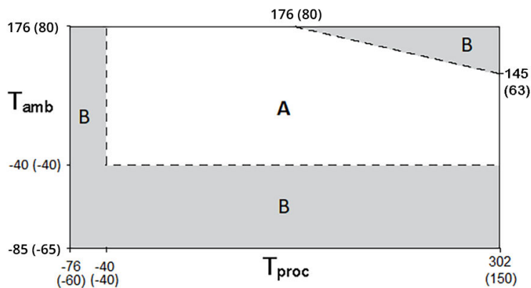
Figura 3: Limites da temperatura do ambiente e do processo para todos os medidores da série G
