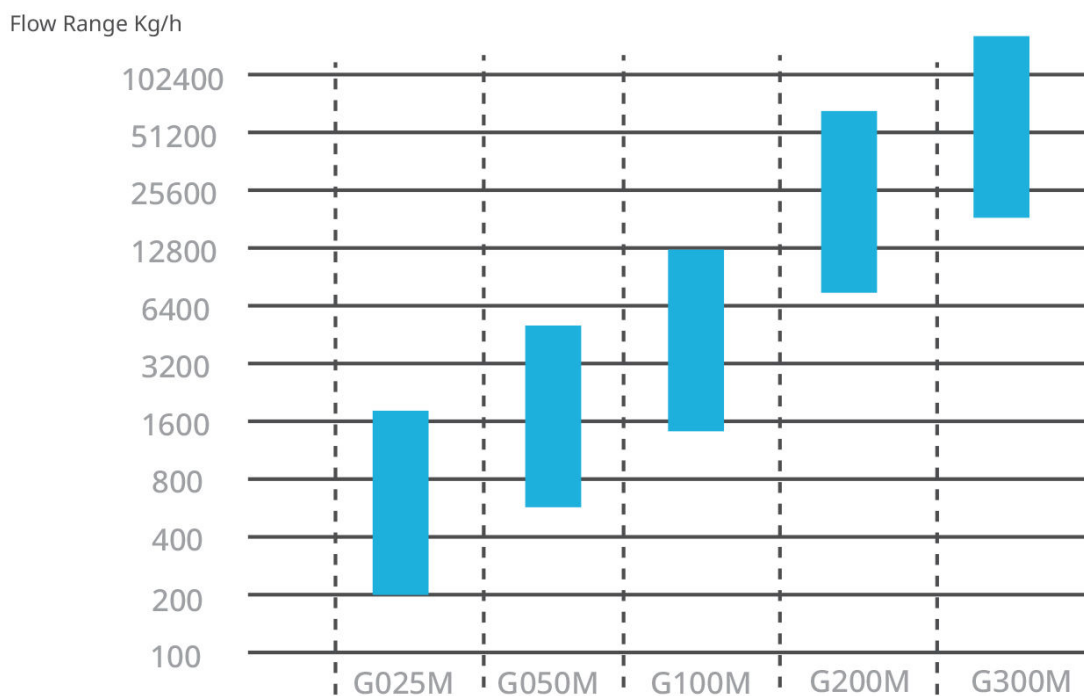
Figura 1: Faixa da medição de vazão e especificações de desempenho da Série G: sistema métrico
