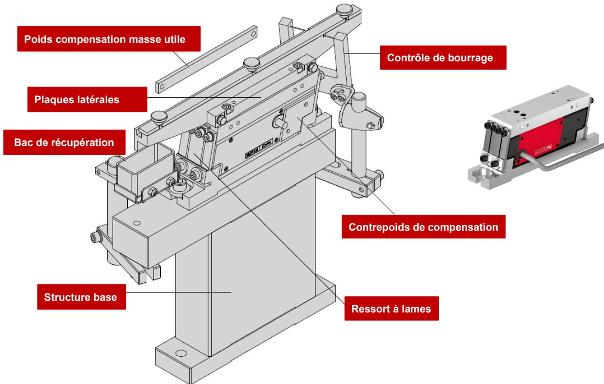
Fig. 3 Structure du HLF-P
