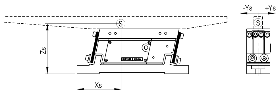
Fig. 5 Zone de la position du centre de gravité (S: Centre de gravité du rail)
