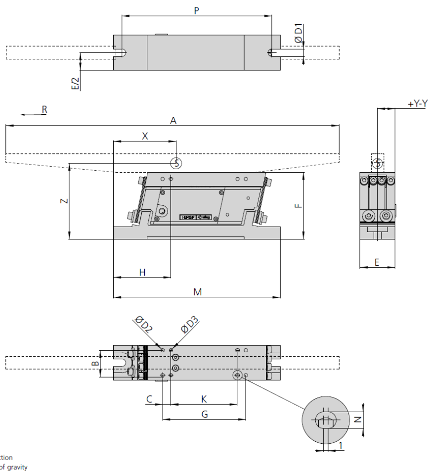
Fig. 1 Schéma coté HLF-P
