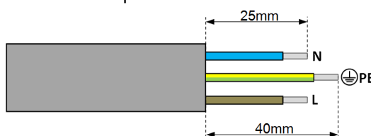
Fig. 8 Extrémité de câble du connecteur supplémentaire
