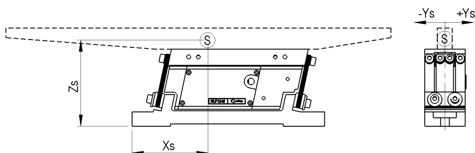
Fig. 10 Zone du centre de gravité - voir aussi Chap. 6.2.3.
