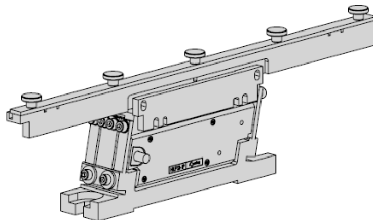
Fig. 7 Montage avec plaque latérale S
