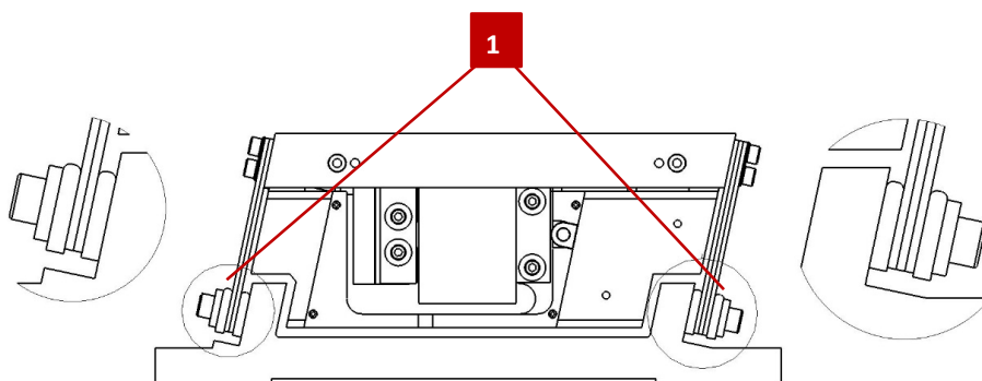
Fig. 11 Ensemble de ressorts avec plaques de réglage
