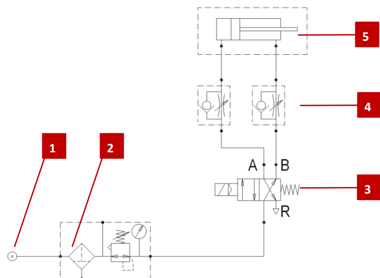
Fig. 15 Schéma du circuit pneumatique chariot compact (4/2)
