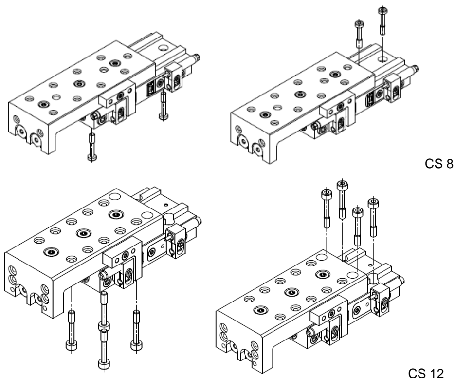
Fig. 13 Montage corps base par bas Montage corps base vissé au travers
