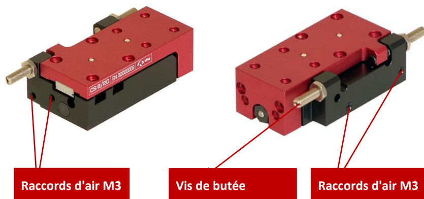
Fig. 19 Mise en service du chariot compact
