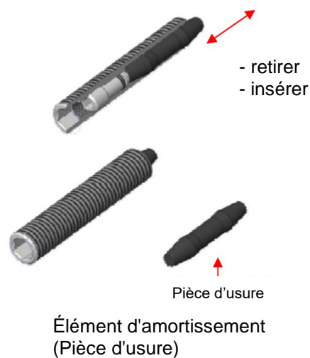
Fig. 21 Remplacement des éléments (amortisseurs en élastomère)
