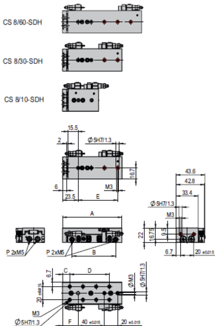
Fig. 2 Schéma coté bras chariot compact CS 8 SDH
