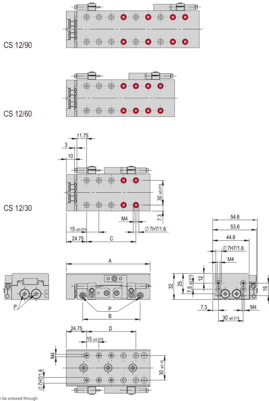
Fig. 6 Schéma coté chariot compact CS 12
