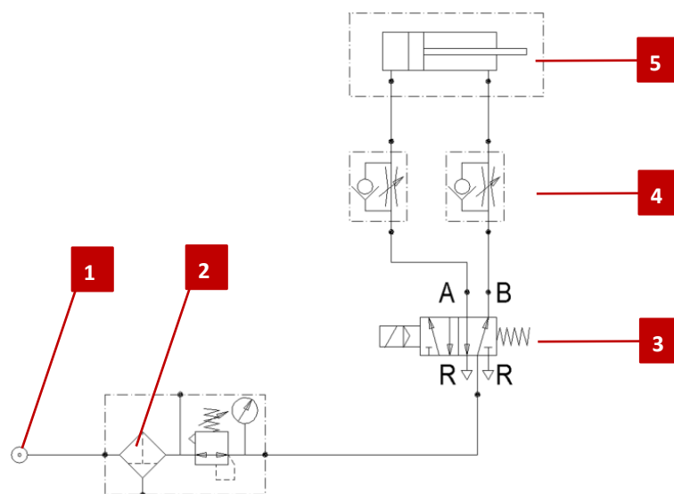
Fig. 14 Schéma du circuit pneumatique chariot compact (5/2)
