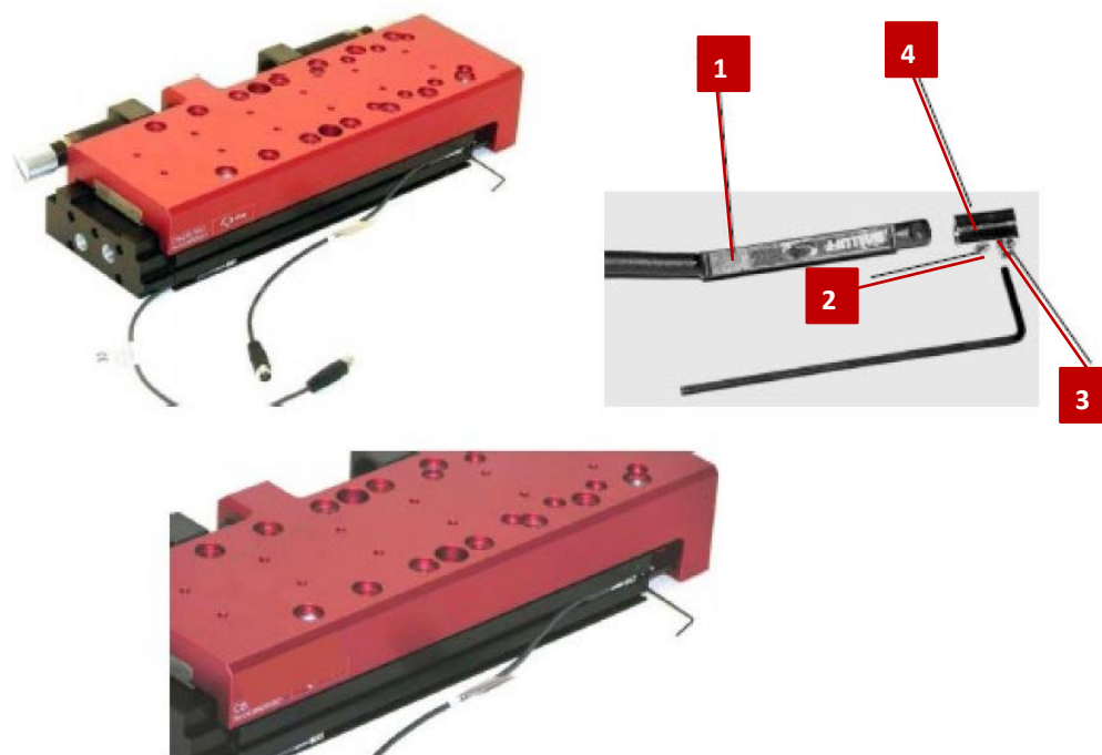
Fig. 16 Installation et réglage du chariot compact
