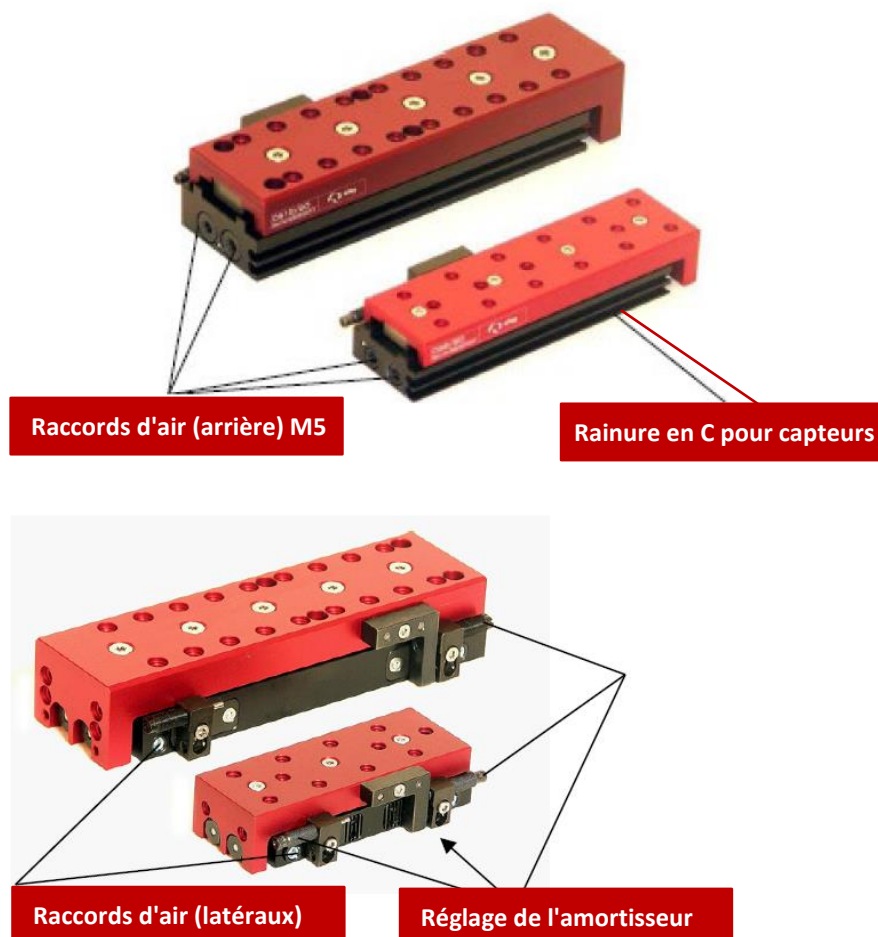
Fig. 18 Réglage des amortisseurs hydraulique
