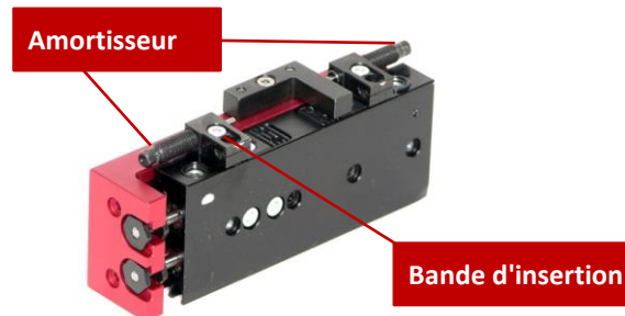
Fig. 17 Réglage des amortisseurs de chocs
