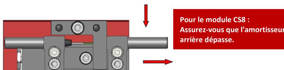
Fig. 18 Réglage des amortisseurs hydraulique
