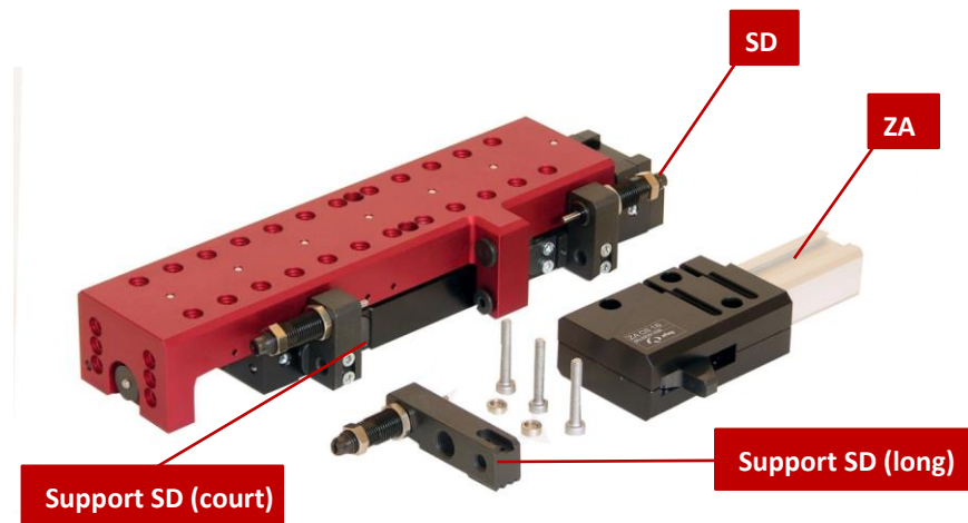
Fig. 21 Montage de la butée intermédiaire ZA
