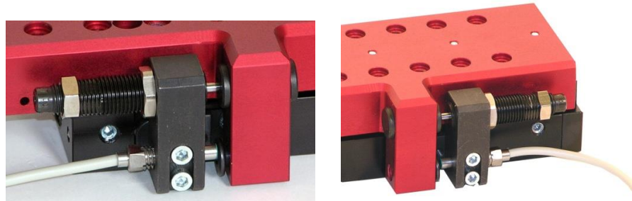
Fig. 18 Capteur (réglable) Détection de la position finale
