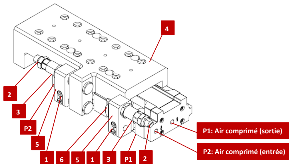
Fig. 26 Installation et réglage du chariot compact
