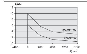
Strømtid diagram (6V/3mW - 8V/22mW) Diagrama do tempo de corrente (6V/3mW - 8V/22mW) Διάγραμμα χρόνου-ρεύματος (6V/3mW - 8V/22mW)
