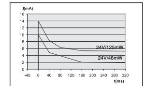
Strømtid diagram (24V/46mW - 24V/125mW) Diagrama do tempo de corrente (24V/46mW - 24V/125mW) Διάγραμμα χρόνου-ρεύματος (24V/46mW - 24V/125mW)
