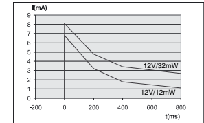
Strømtid diagram (12V/12mW - 12V/32mW) Diagrama do tempo de corrente (12V/12mW - 12V/32mW) Διάγραμμα χρόνου-ρεύματος (12V/12mW - 12V/32mW)
