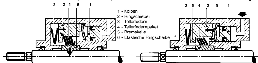
DRUCKLOS: Klemmung der Kolbenstange
