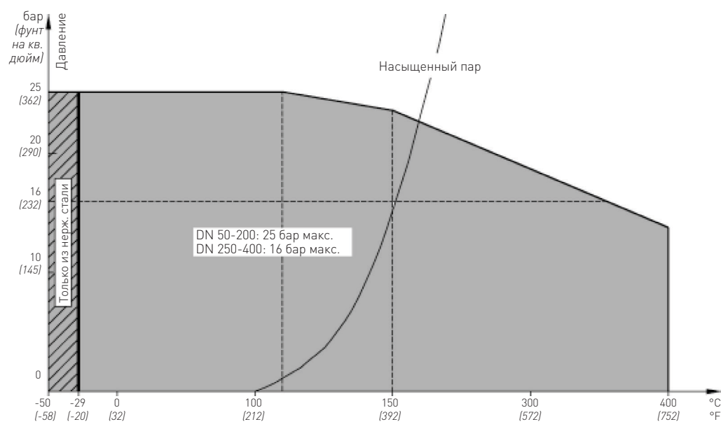
ДИАГРАММА Р/Т (ДАВЛЕНИЕ/ТЕМПЕРАТУРА) (НИЛОК НТ СЕДЛО)
