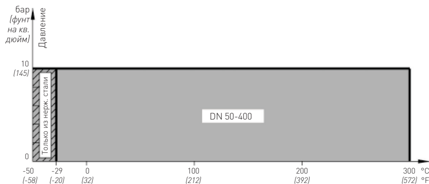
ДИАГРАММА Р/Т (ДАВЛЕНИЕ/ТЕМПЕРАТУРА) (НИЛОК РР СЕДЛО)
