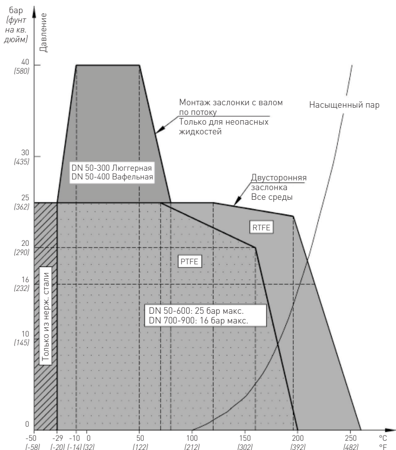
ДИАГРАММА Р/Т (ДАВЛЕНИЕ/ТЕМПЕРАТУРА) (HILOK УСИЛЕННЫЙ ТЕФЛОН И ОГНЕСТОЙКОЕ)
