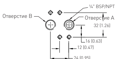
Размеры присоединения воздуха 002 - 052
