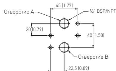
Размер присоединения воздуха 240
