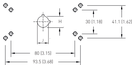
Размеры верхних крепежных отверстий 032 - 052
