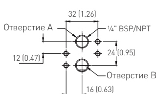
Размеры присоединения воздуха 085 - 140
