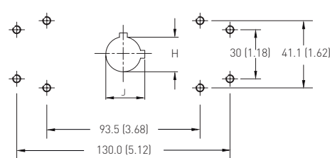
Размеры верхних крепежных отверстий 084 - 240
